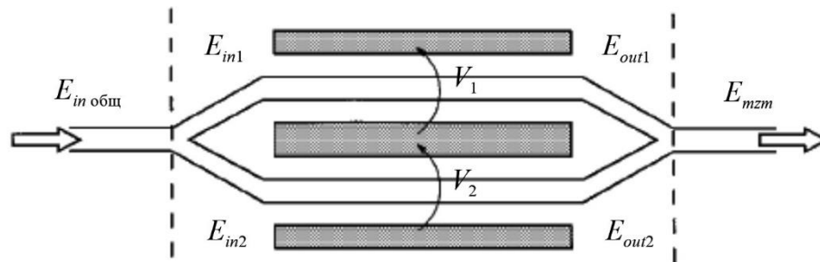
Рис. 3. Структурная схема двухпортового ДПММЦ [15]
