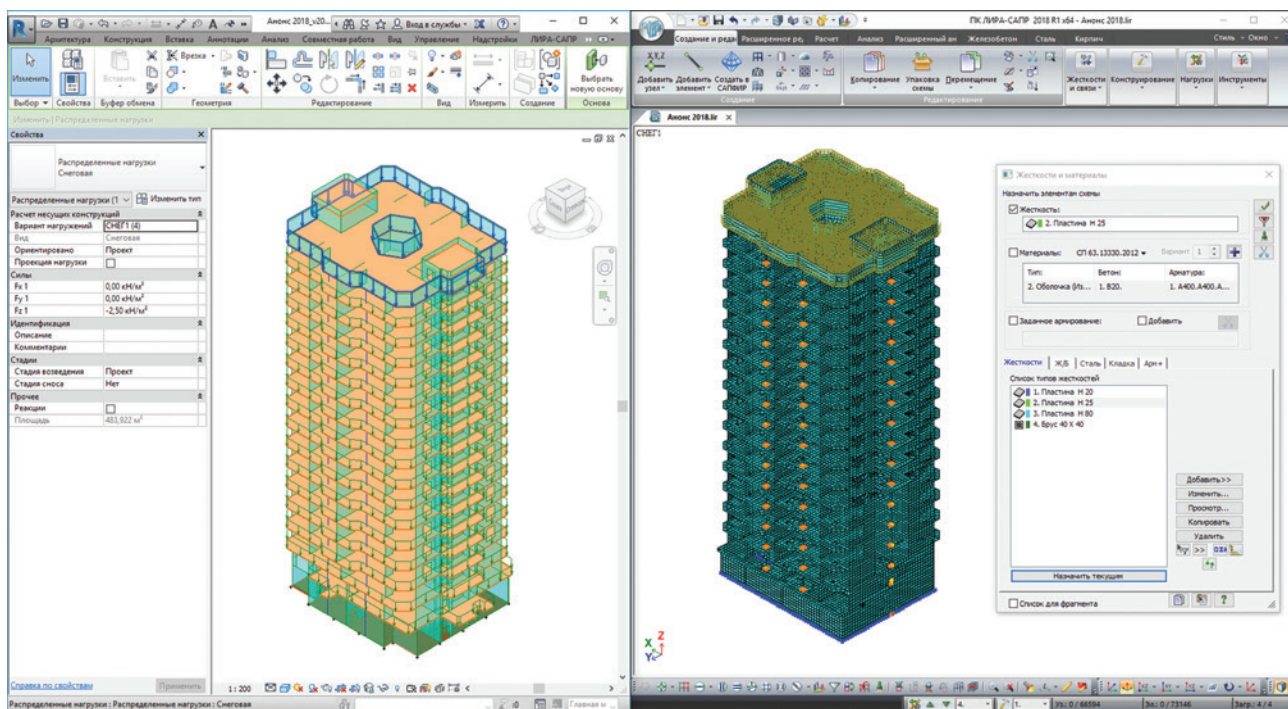
Рис. 1. Аналитическая модель, созданная в Revit и импортированная в Lira
