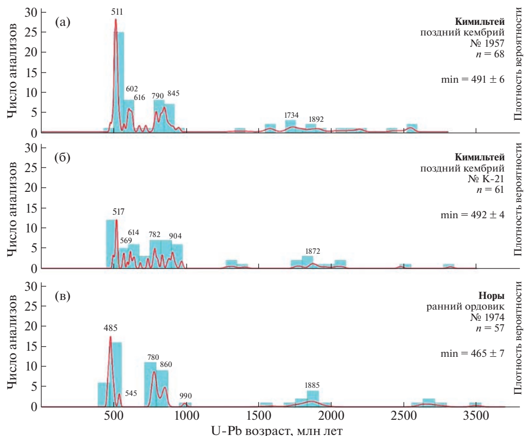
Рис. 3. Гистограммы и кривые плотности вероятности возрастов зерен детритового циркона из проб разреза Кимильтей № 1957 (а), № К21 (б) и разреза Норы № 1974 (в).
