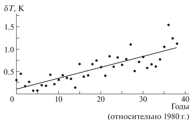
Рис. 2. Аномалии (относительно базового периода 1961–1990 гг.) зимней приповерхностной температуры СП T [K] в СП в зависимости от времени t (годы относительно 1980 г.) для периода 1980–2018 гг. Прямая линия соответствует линейной регрессии.
