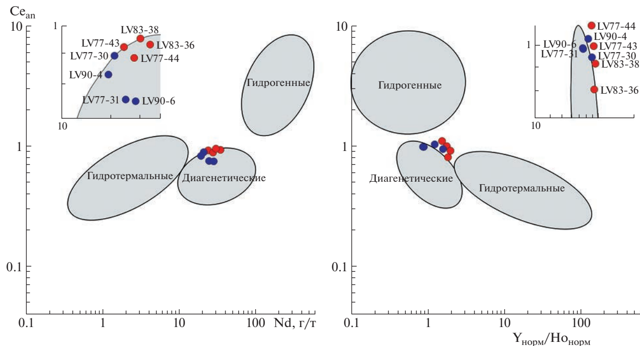
Рис. 4. Положение ЖМО ВСМ относительно полей разных генетических типов ЖМО океана на диаграммах М. Бай [3] в общем и укрупненном виде. Красные кружки – ЮЗ-район, синие – СЗ-район. Краткая характеристика образцов дана в примечании к табл. 1.
