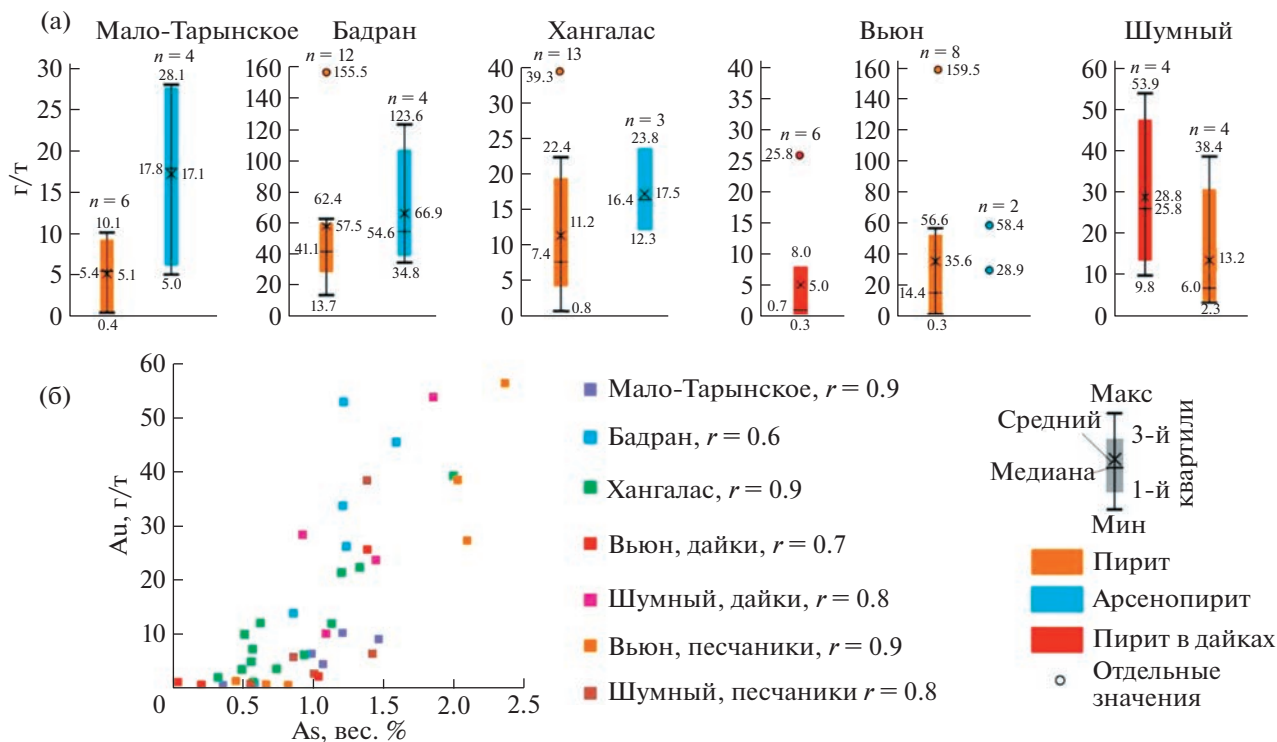
Рис. 3. Содержание золота в сульфидах из метасоматитов изученных месторождений (а) и диаграмма соотношения между концентрациями As и Au в Py3 (б).
