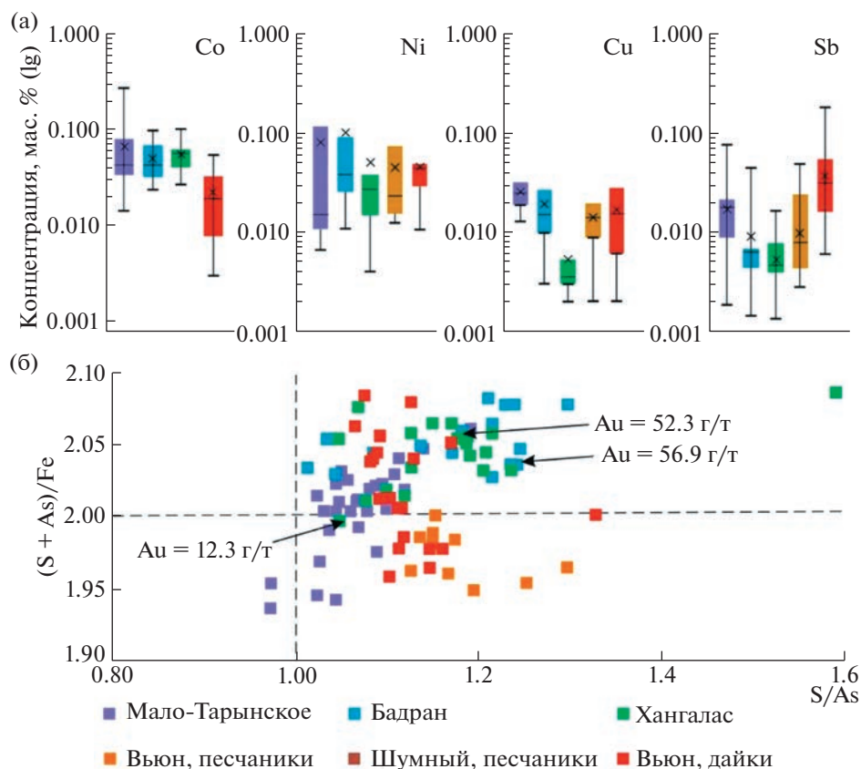
Рис. 4. Распределение элементов-примесей в арсенопирите (а) из метасоматитов и диаграмма соотношений S/As и (S + As)/Fe (б) изученных месторождений ЯКМП. Пересечение линий S/As = 1 и (S + As)/Fe = 2 соответствует стехиометрическому составу [13].
