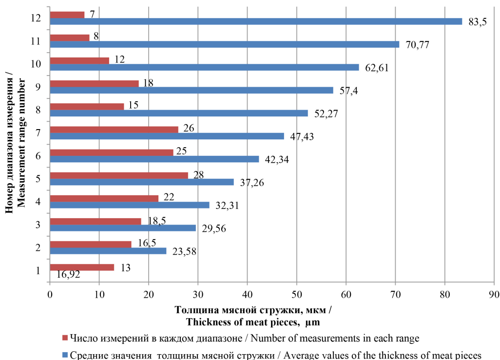
Р и с. 1. Гистограмма распределения размера (толщины) мясной стружки при одностадийном измельчении. Диапазоны измерения: 1 – 14–20 \mu\text{m} ; 2 – 20–26 \mu\text{m} ; 3 – 26–30 \mu\text{m} ; 4 – 30–35 \mu\text{m} ; 5 – 35–40 \mu\text{m} ; 6 – 40–45 \mu\text{m} ; 7 – 45–50 \mu\text{m} ; 8 – 50–55 \mu\text{m} ; 9 – 55–60 \mu\text{m} ; 10 – 60–66 \mu\text{m} ; 11 – 66–76 \mu\text{m} ; 12 – 76–91 \mu\text{m}
