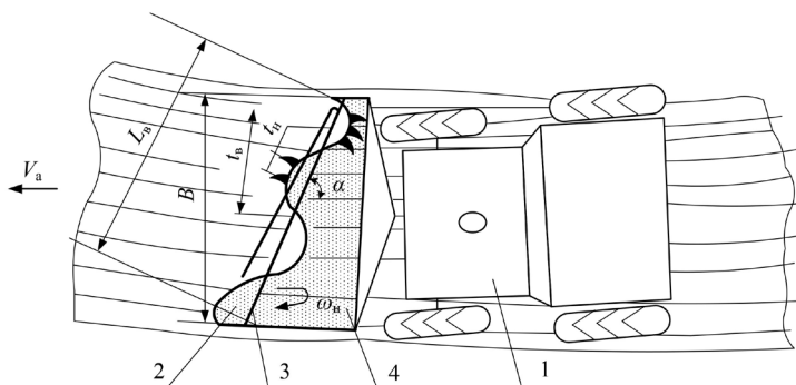
Р и с. 7. Схема агрегата: 1 – энергетическое средство; 2 – винт измельчителя; 3 – вал винта; 4 – стеблестой; L_a – длина вала винта; t_e – шаг винтов; t_n – шаг ножей; B – ширина захвата; \alpha – угол атаки; \omega_n – угловая скорость ножей
