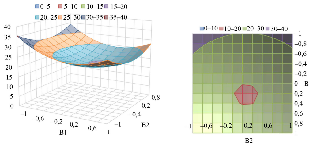
Р и с. 12. Графическое место точек для зависимости \gamma_2 = f(\beta_1; \beta_2; \beta_3 = 0) \rightarrow \min F i g. 12. Graphical location of points for the dependence \gamma_2 = f(\beta_1; \beta_2; \beta_3 = 0) \rightarrow \min
