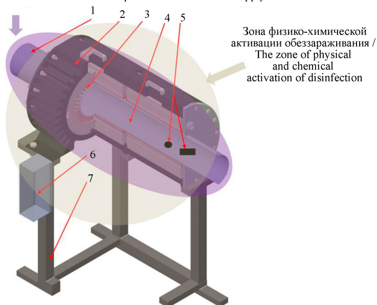
Р и с. 1. Общий вид активатора обеззараживания в разрезе:
