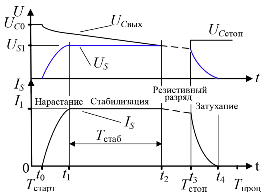
Р и с. 5. Графики, поясняющие работу схемы питания на примере одного канала
