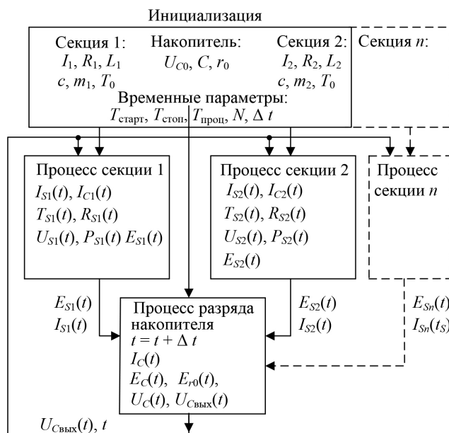
Р и с. 6. Блок-схема математической модели
