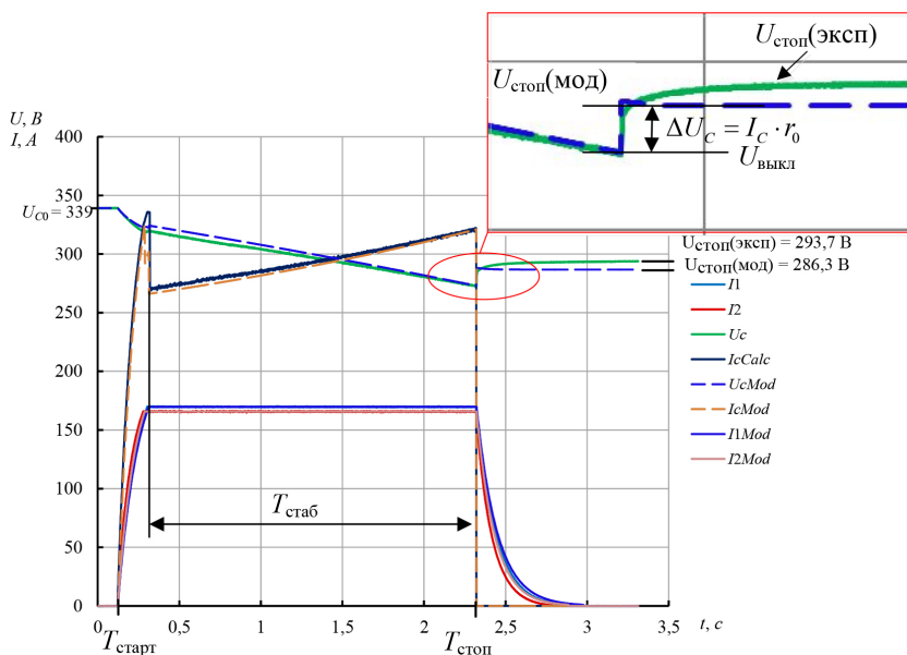
Р и с. 7. Форма выходного тока и напряжения накопителя по результатам эксперимента и моделирования: I_1 , I_2 , U_c – экспериментальные формы тока и напряжения; IcCalc – расчетный выходной ток накопителя; UcMod , IcMod , I1Mod , I2Mod – результаты моделирования
