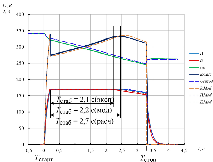
Р и с. 8. Форма тока и напряжения при максимальной длительности стабилизации тока
