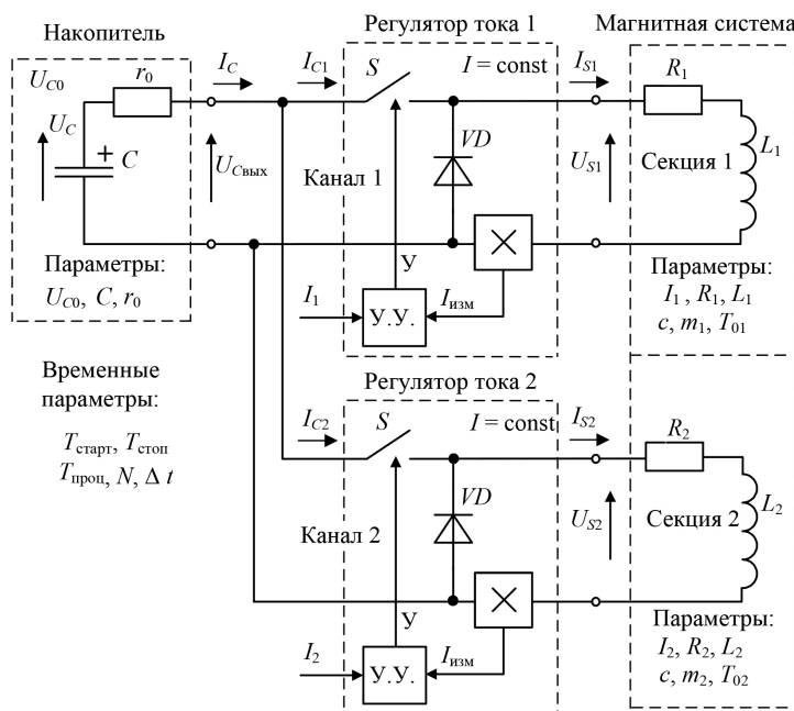
Р и с. 4. Схема питания двухсекционной магнитной системы от суперконденсаторного накопителя
