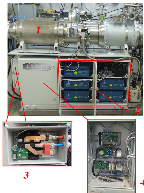
Р и с. 2. Внешний вид магнитной системы с источником питания: 1 – магнитная система; 2 – накопитель; 3 – регуляторы тока; 4 – контроллер с элементами схемы зарядки и разрядки Fig. 2. Appearance of magnetic system with its power supply: 1 – magnetic system; 2 – supercapacitor storage; 3 – current regulators; 4 – controller with parts of charging and discharging circuit
