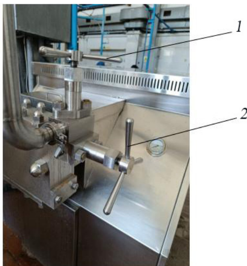
Р и с. 1. Гомогенизатор. Узел регулировки давления: 1 – винт второй ступени; 2 – винт первой ступени F i g. 1. The homogenizer. Pressure control unit: 1 – second stage screw; 2 – first stage screw
