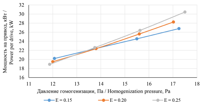
Р и с. 3. Зависимость мощности на привод гомогенизатора N от давления P F i g. 3. Dependence of the drive power of the homogenizer N on the pressure P
