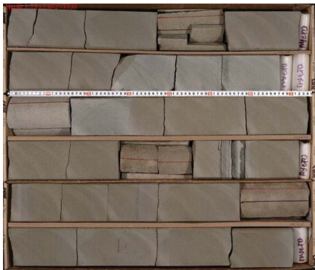
Рис. 10. Тестовая фотография ядра Fig. 10. Core test photo
