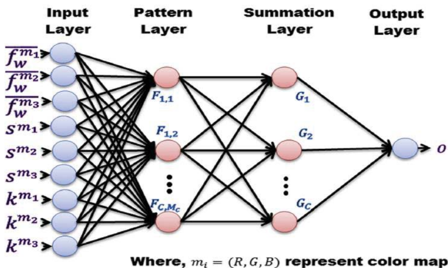
Рис. 1. Архитектура PNN
