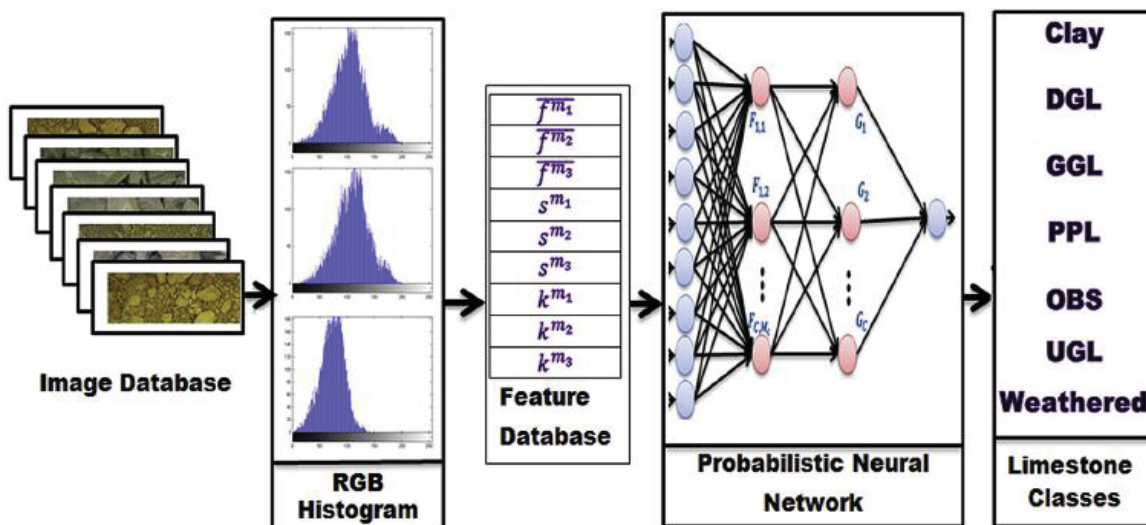
Рис. 2. Методология классификации
