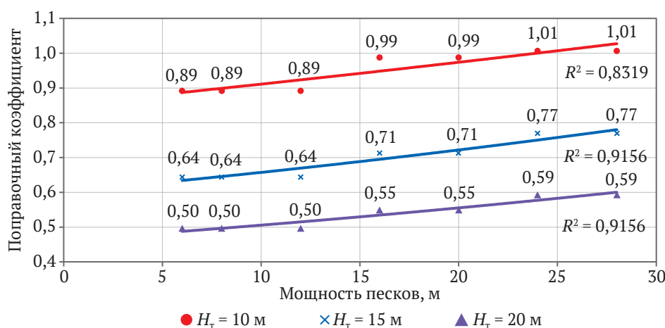
Рис. 7. Зависимости поправочного коэффициента от параметров россыпи при бестранспортном способе производства вскрышных пород и мощности торфов 10, 15, 20 м
