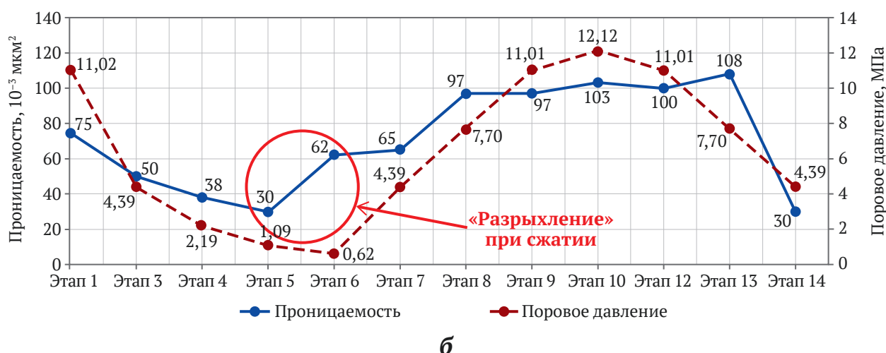
Рис. 5. Результаты лабораторных исследований для образца 6, насыщенного керосином с остаточной водой: а – изменение модуля Юнга, б – изменение проницаемости по этапам эксперимента. Красной штриховой линией показано изменение порового давления
