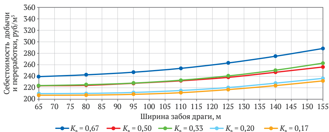
Рис. 4. Зависимости себестоимости добычи и переработки полезного ископаемого от ширины дражного забоя при мощности торфов 4 м и коэффициенте вскрыши K_b = 0,17–0,67
