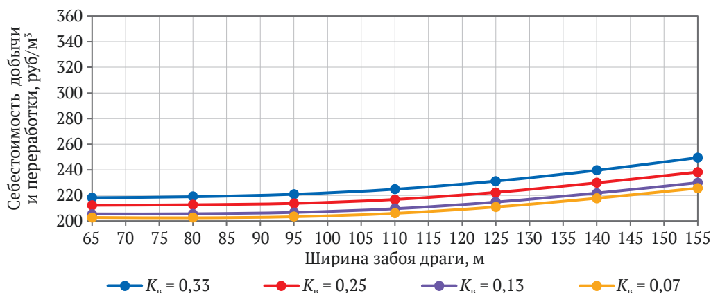
Рис. 3. Зависимости себестоимости добычи и переработки полезного ископаемого от ширины дражного забоя при мощности торфов 2 м и коэффициенте вскрыши K_b = 0,07–0,33
