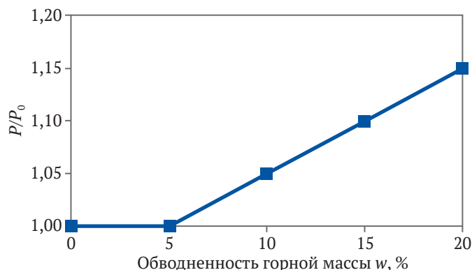
Рис. 4. Зависимость отношения P/P_0 от степени обводненности просыпанной горной массы w
