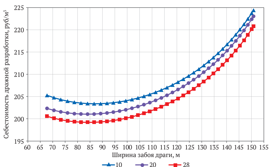
Рис. 2. Зависимости себестоимости драгирования от ширины забоя для 380 л драги при мощности продуктивного пласта 10, 20, 28 м
