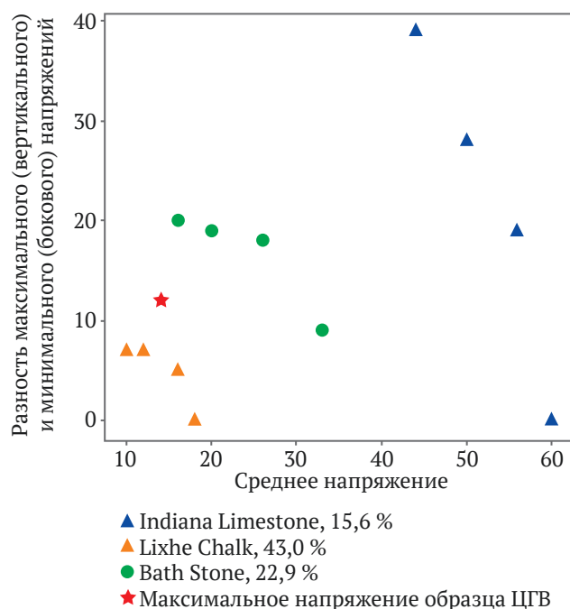
Рис. 6. Огибающие разрушения сжатия по данным работы [8] и предельное напряженное состояние для образца турнейского яруса
