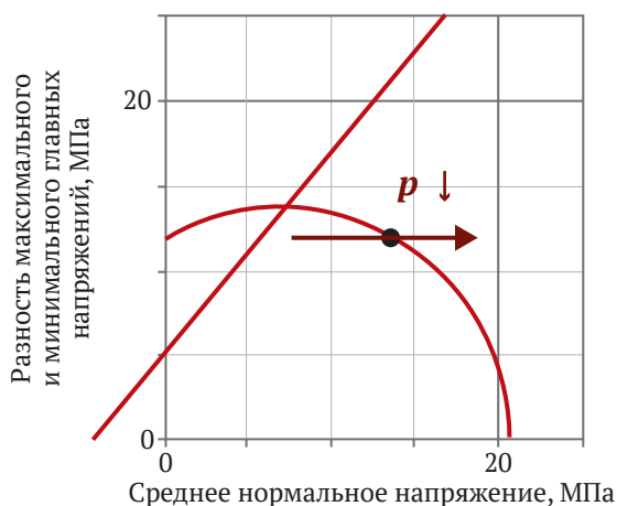
Рис. 9. Огибающая для критерия разрушения сжатия и точка срабатывания критерия, полученная экспериментально, а также прямая Мора–Кулона для разрушения сдвига
