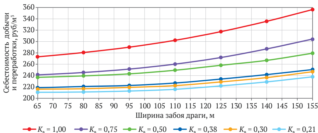
Рис. 5. Зависимости себестоимости добычи и переработки полезного ископаемого от ширины дражного забоя при мощности торфов 6 м и коэффициенте вскрыши K_b = 0,21–1,00
