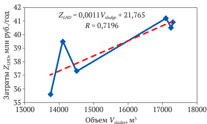
Рис. 5. Зависимость затрат на ремонты погрузочно-доставочных машин Z_{LHD} от объема перевозимых ими продуктов заиливания за год V_{sludge}
