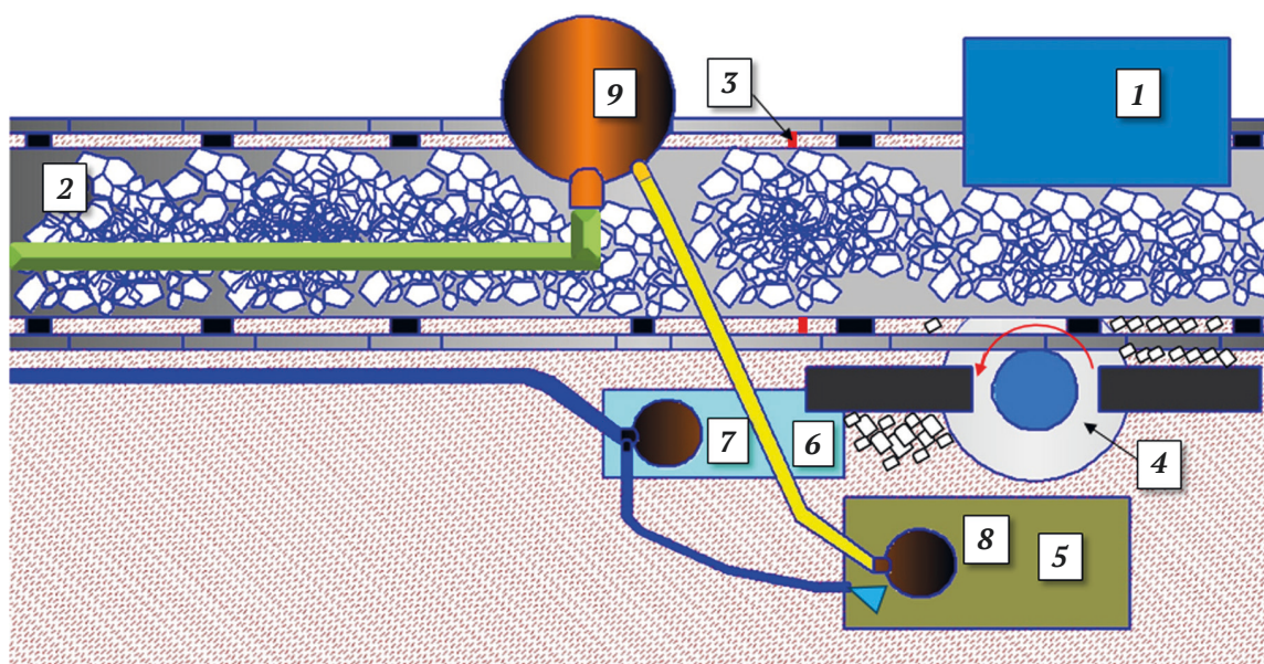
Рис. 2. Механизированный комплекс по сбору просыпанной руды: 1 – питатель; 2 – ленточный конвейер; 3 – перегородка; 4 – заборно-погрузочное устройство; 5 – шламособорник; 6 – водособорник; 7 – погружной насос; 8 – погружной насос с агитатором; 9 – емкость для сбора приготовленной пульпы
