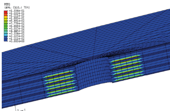
Рис. 8. Численное решение задачи о распределении напряжений в окрестности перфорационных каналов при плотности перфорации 8 перфорационных отверстий на 0,3 м для обсаженной скважины. Синим цветом показана зона упругости, другими цветами – зона срабатывания критерия сдвигового разрушения [15]
