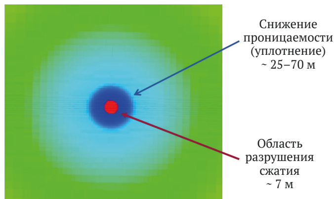
Рис. 10. Поле коэффициента изменения проницаемости по результатам расчетов сопряженной модели в tNavigator (гидродинамика + геомеханика) с использованием скрипта для учета уплотнения и разрушения сжатия через анализ эффективных напряжений. Цвета пояснены в тексте
