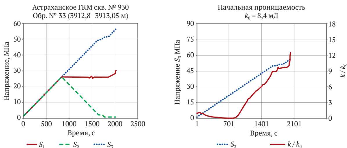
Рис. 2. Этапы нагружения и изменение проницаемости карбонатного образца (Астраханское месторождение) Источник: Коваленко Ю. Ф. Геомеханика нефтяных и газовых скважин. [Дис. ... д-ра физ.-мат. наук]. М., 2012. 314 с.
