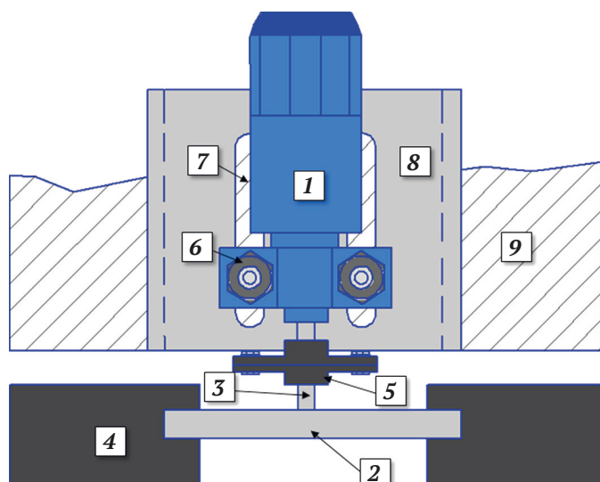
Рис. 3. Заборно-погрузочное устройство:
