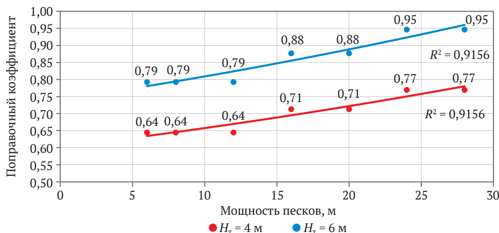
Рис. 6. Зависимости поправочного коэффициента от параметров россыпи при бульдозерном способе производства вскрышных пород при мощности торфов 4 и 6 м
