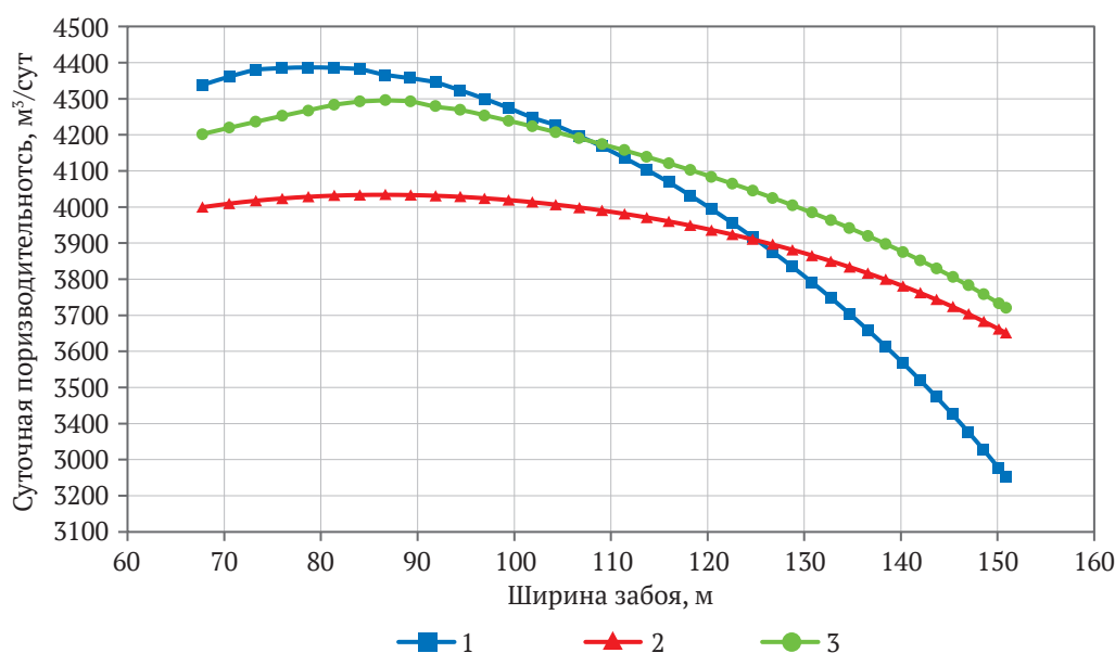
Рис. 1. Зависимости суточной производительности 380 л драги от ширины забоя: 1 – по методике В.А. Кудряшева; 2 – по методике В.Г. Лешкова; 3 – по методике С.М. Шорохова
