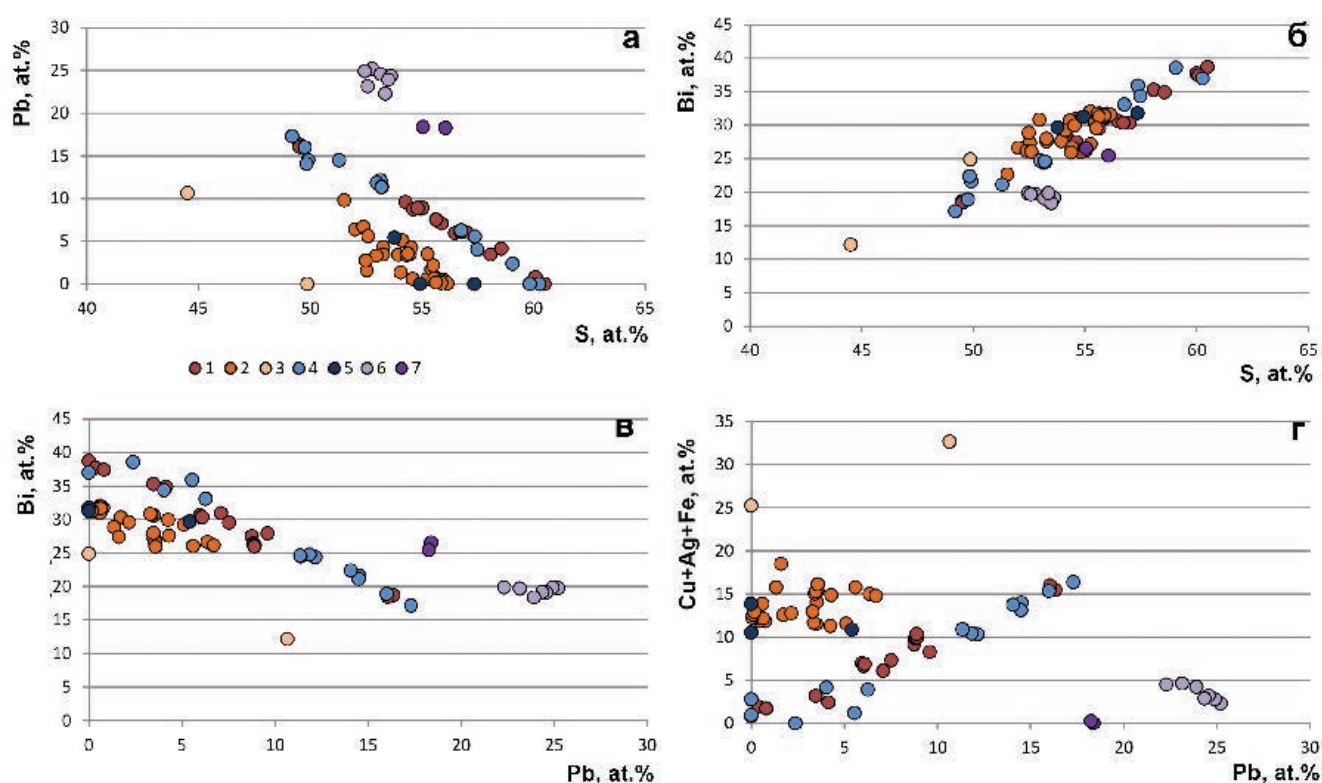
Рис. 7. Бинарные диаграммы, демонстрирующие разнообразие химических составов висмутовых сульфосолей Юго-Коневского (1–3) и Пороховского (4–7) месторождений.
