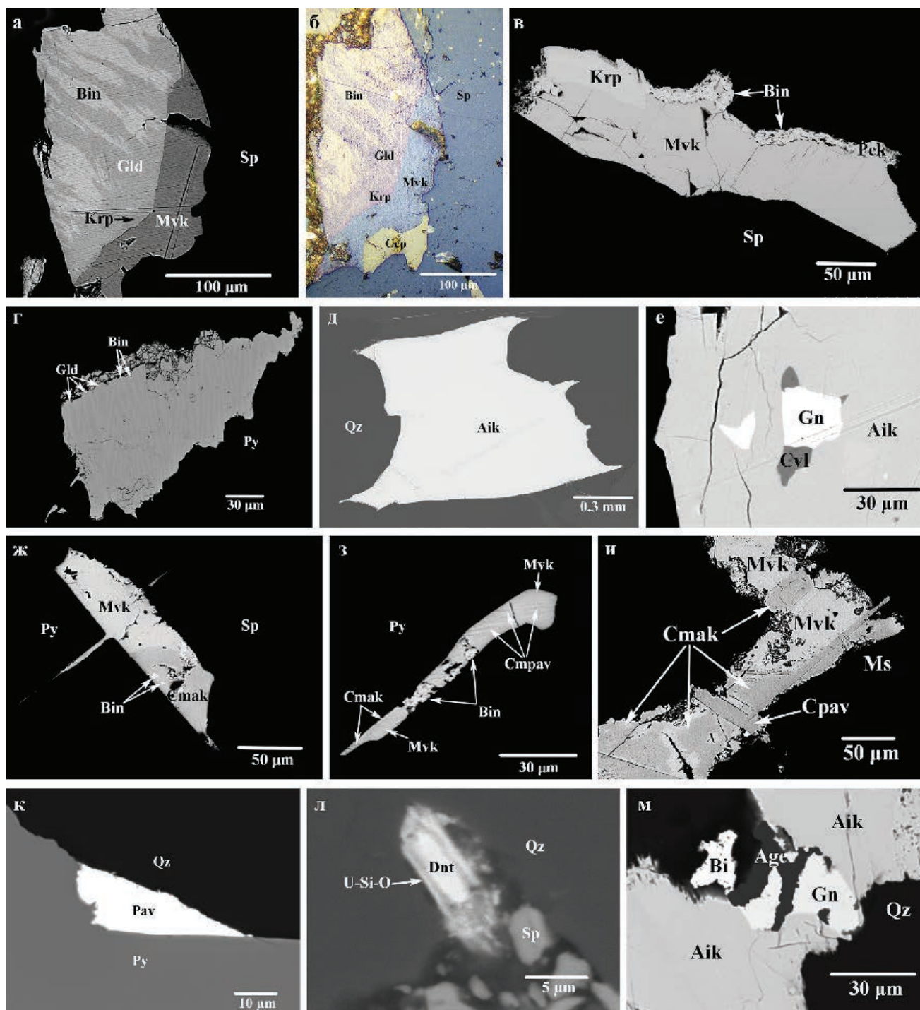
Рис. 4. Морфология сульфосалей Юго-Коневского месторождения: а – сросток висмута (Bin), гладиита (Gld), крупкаита (Krp) и маковицкиита (Mvk) с халькопиритом (Ccp) в сфалерите (Sp); б – тот же сросток в отраженном свете, николи частично скрещены; в – сросток висмута, пекоита (Pek), крупкаита и маковицкиита в сфалерите; г – структура распада висмутин-гладиитового состава в пирите (Py); д – крупное зерно айкинита (Aik) в кварце (Qz); е – включения галенита (Gn) и сервеллеита (Cvl) в айкинита; ж – сросток маковицкиита и купромаковицкиита (Cmak) на контакте пирита и сфалерита, в купромаковицкиите – мелкие включения висмута; з – тонкие ламели купромакопавонита (Cmpav) и купромаковицкиита (более темные на фото) в маковицкиите (более светлый) с висмутином в пирите; и – сросток маковицкиита, купромаковицкиита и купропавонита (Cpav) в мусковите (Ms); к – зерно павонита (Pav) на контакте пирита и кварца; л – зерно дантопайта с каймой неуставленного уранилсиликата (U-Si-O) в кварце со сфалеритом; м – прожилки ангелайта (Age) в галените с айкинитом и висмутом (Bi) в кварцевой вмещающей породе.
