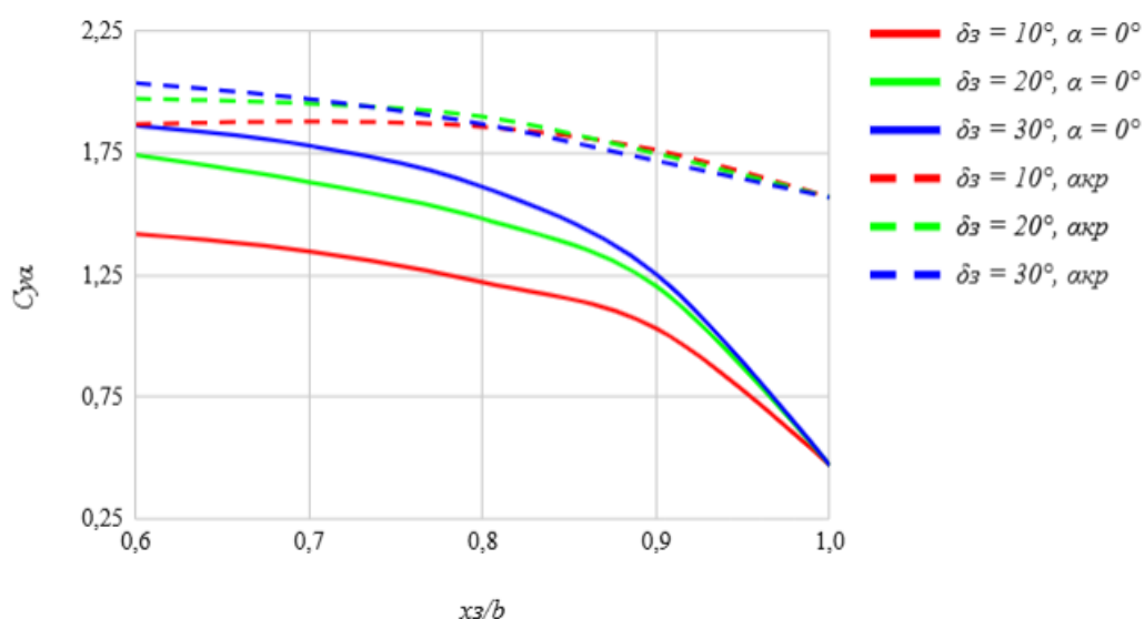
Рисунок 7 – Зависимость C_{y\alpha} = f(x_3 / b) для простого и адаптивного закрылков при \alpha = 0^\circ и \alpha_{кр} при \delta_6 = 10...30^\circ
