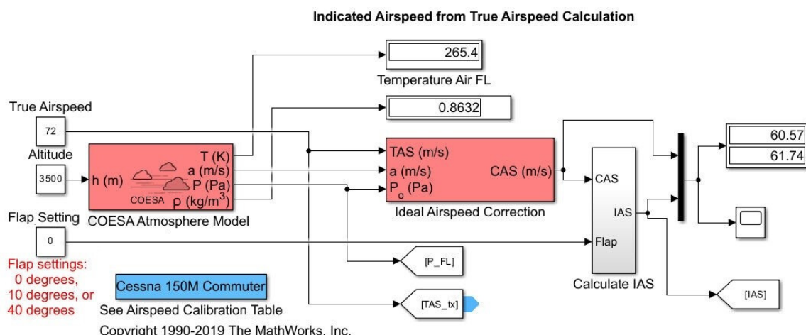
Рисунок 2 – Модель Simulink
