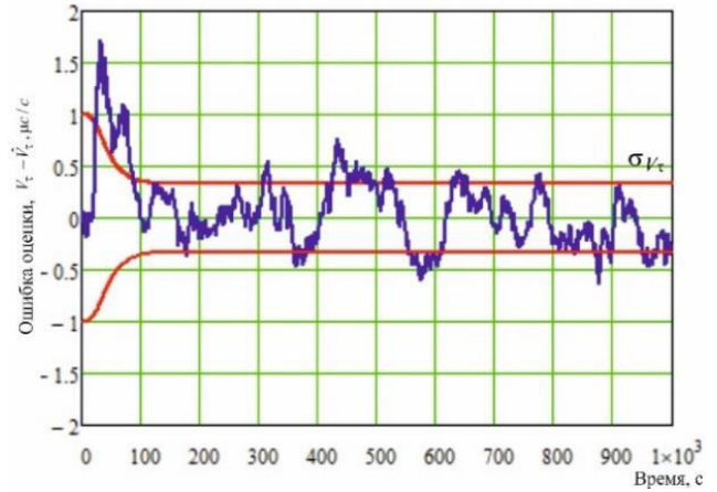
Рисунок 2 – Ошибка оценки скорости изменения времени задержки
