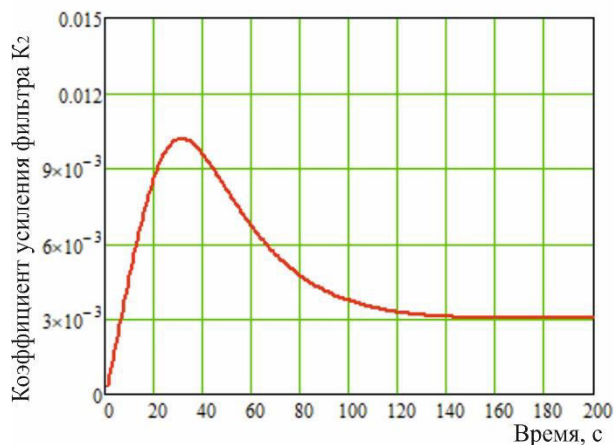
Рисунок 8 – Коэффициент усиления фильтра K_{2,v}
