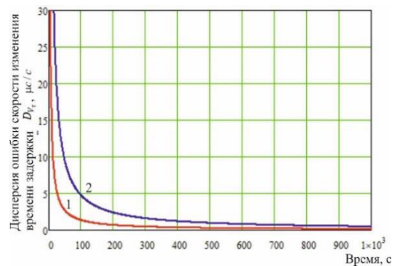
Рисунок 6 – Дисперсия ошибки оценки скорости изменения времени задержки: 1 – при корректной работе; 2 – при расходимости.
