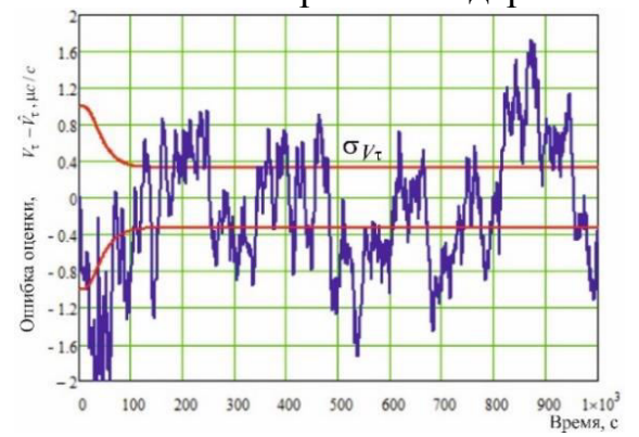
Рисунок 4 – Ошибка оценки скорости изменения времени задержки при расходимости
