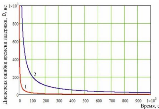
Рисунок 5 – Дисперсия ошибки оценки времени задержки: 1 – при корректной работе; 2 – при расходимости.
