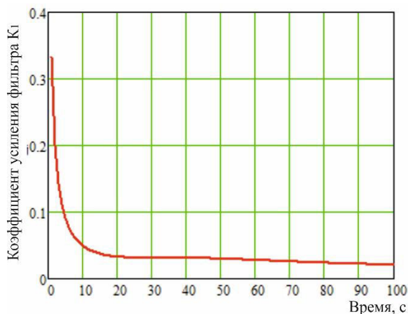
Рисунок 7 – Коэффициент усиления фильтра K_{1,v}
