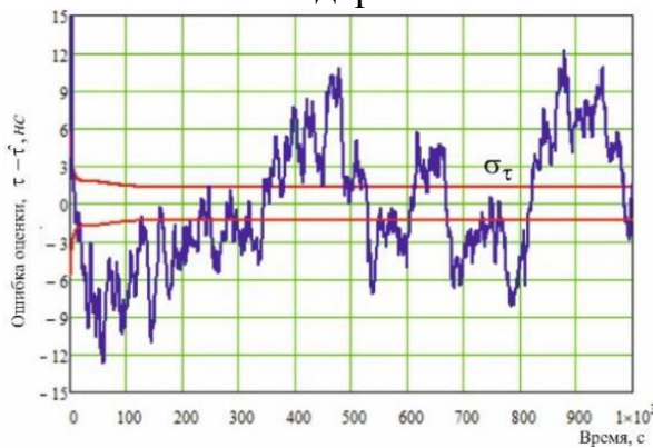
Рисунок 3 – Ошибка оценки времени задержки при расходимости
