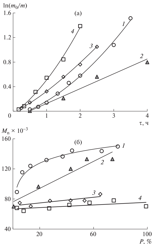
Рис. 3. Зависимости \ln(m_0/m) MMA от времени синтеза (а) и M_n ПММА от конверсии мономера (б) при облучении белым светом. Молярное соотношение MMA : ЭБИБ : метиленовый синий : амин = 100 : 1 : 0.01 : 0 (1), 100 : 1 : 0.01 : 5 (2) и 100 : 1 : 0.01 : 0.5 (3, 4). Амины: 1 — без введения амина, 2 — i\text{-PrNH}_2 , 3 — ПМДЭТА, 4 — \text{Et}_3\text{N} .
