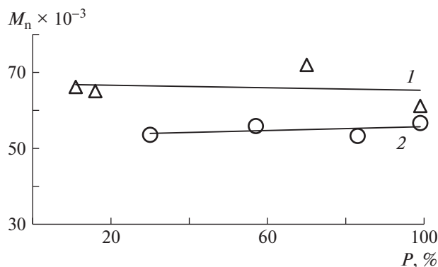
Рис. 2. Зависимость M_n ПММА от конверсии мономера при облучении светом \lambda_{max} = 365 нм. Молярное соотношение MMA : ЭБИБ : метиленовый синий : аскорбиновая кислота = 100 : 1 : 0.01 : 5 (1) и 100 : 1 : 0.1 : 5 (2).
