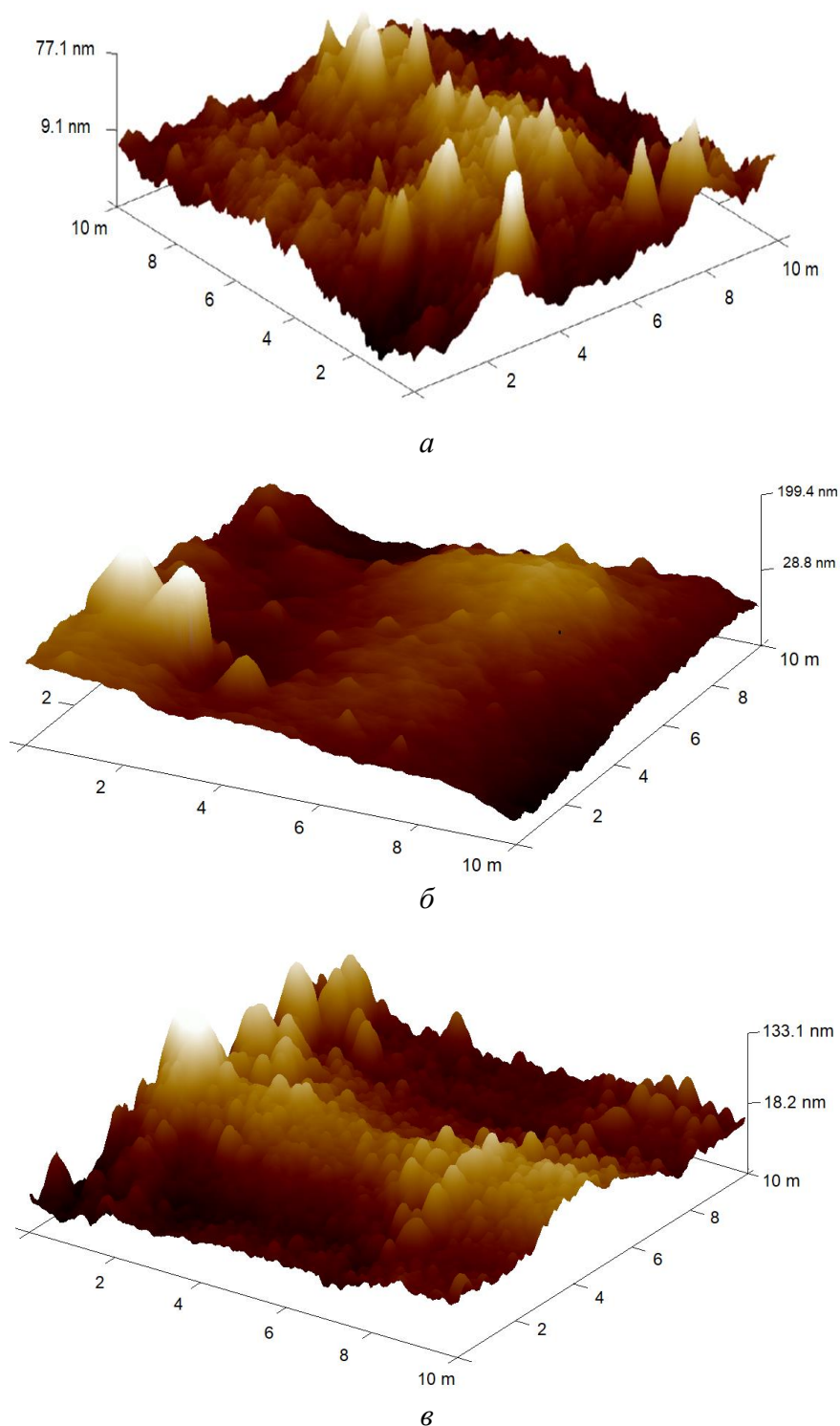
Рис. 4. АСМ-изображение топографической поверхности исходного ПП образца ( a ), активированных в средах аргона ( б ) и в аргон – воздух в соотношении 50:50 ( в )
