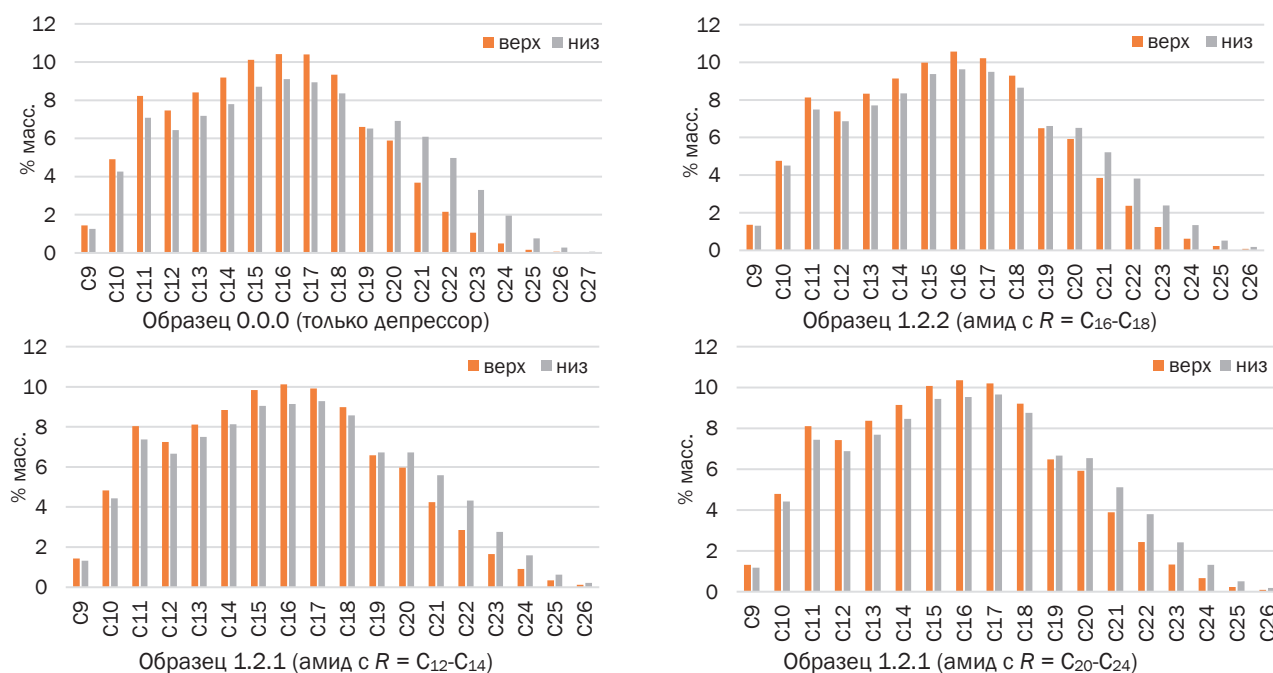
Рис. 3. Молекулярно-массовое распределение n -алканов в верхнем и нижнем слоях испытуемых образцов дизельного топлива 2
