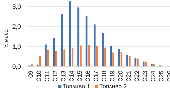
Рис. 1. Молекулярно-массовое распределение n -алканов в испытуемых дизельных топливах 1 и 2
