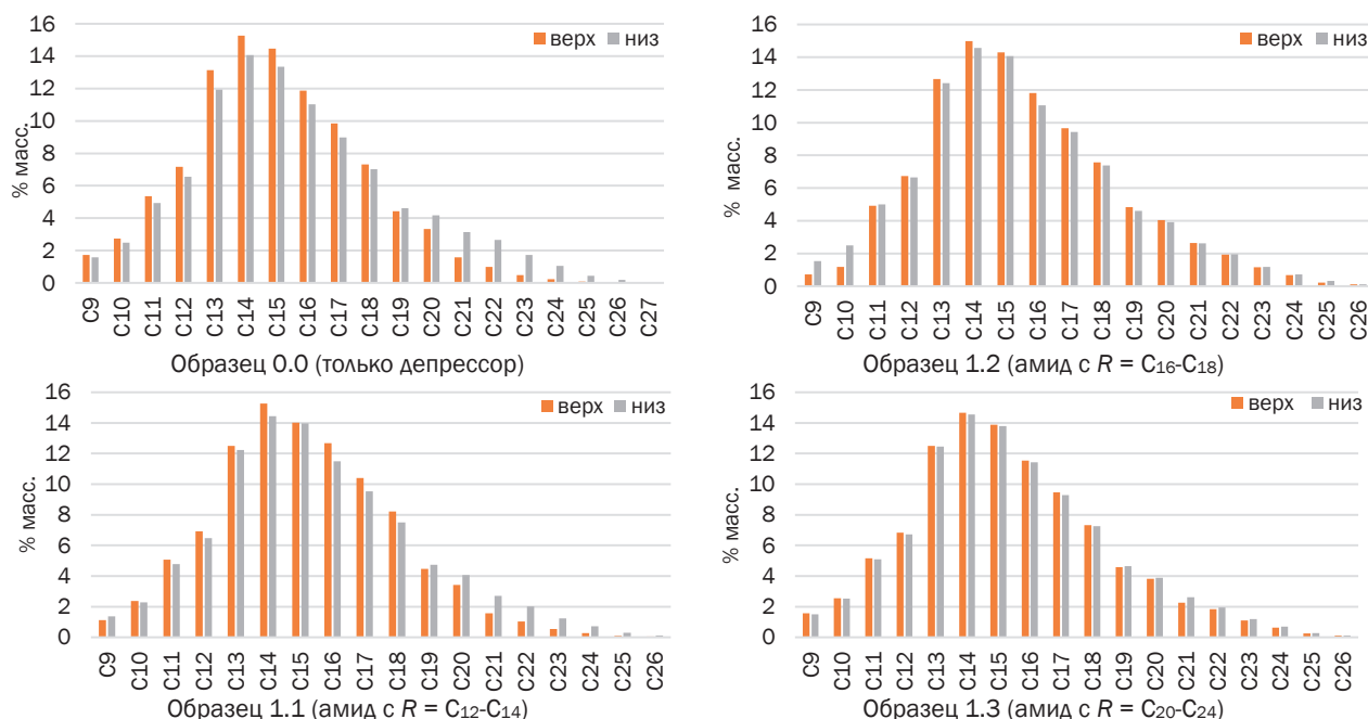
Рис. 2. Молекулярно-массовое распределение n -алканов в верхнем и нижнем слоях испытуемых образцов дизельного топлива 1
