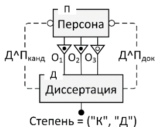
Рисунок 8 – Пример расщеплённого МП-ограничения
