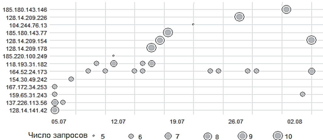
Рисунок 5 – Пример статистики нелегитимных обращений (оси: дата, ip -адрес источника обращения)
