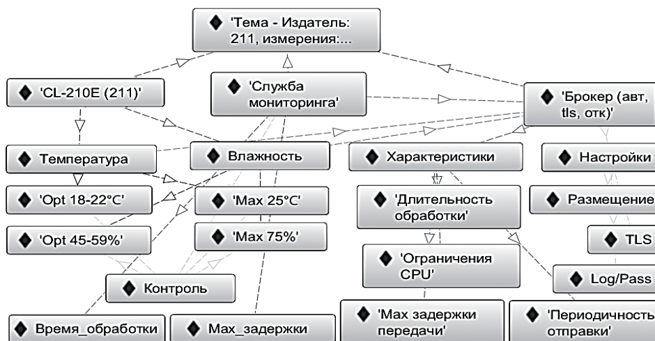
Рисунок 3 – Фрагмент графического представления экземпляров классов
