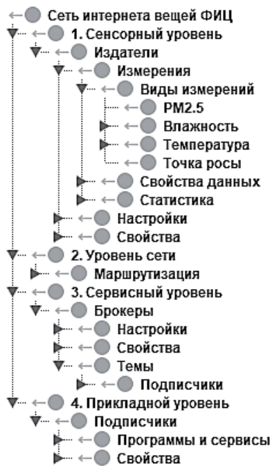
Рисунок 1 – Иерархическая структура классов
