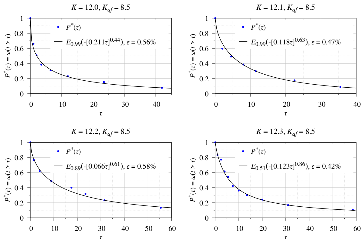
Рис. 2. График эмпирического закона P^*(\tau) распределения времени ожидания афтершоков и его аппроксимация функцией Миттаг–Леффлёра E_\nu(-[\mu\tau]^\nu) (1).
