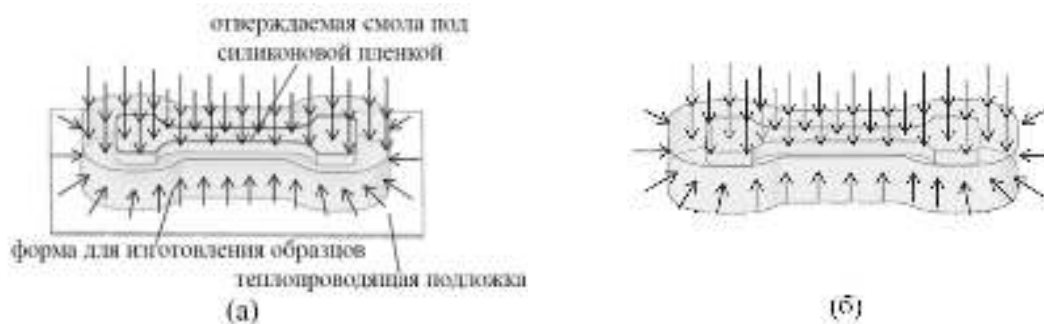
Рис. 2. Схематичное представление образца связующего ВСТ-1208, налитого в силиконовую форму, в условиях прогрева: а) в вакуумном термошкафу на теплопроводящей подложке и б) в вакуумном термошкафу без теплопроводящей подложки
