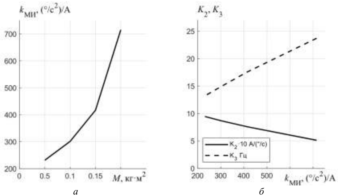
Рис. 8. а – коэффициент k_{MH} , б – коэффициенты K_2 и K_3 регулятора контура скорости
