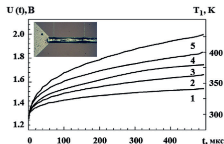
Рис. 6. Осциллограммы включения системы Si-Ti-Al при различной толщине подслоя Ti: 1 – h_2=0 ; 2 – h_2=80 ; 3 – h_2=100 ; 4 – h_2=130 ; 5 – h_2=170 нм; j=6.0 \cdot 10^{10} А/м 2 ; h_1=2 мкм; длительность импульсов 500 мкс. На вставке: фотография структуры Al-Ti-Si после прохождения импульса тока j > j_{кр} .
