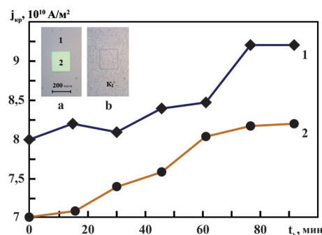
Рис. 7. Зависимость величины критической плотности тока j_{кр} от времени отжига t_h структуры Al-Ti-Si в инертной атмосфере при температуре 500 °C; длительность прямоугольного импульса тока: 1 – 550 мкс; 2 – 200 мкс. На вставке: микрофотографии многослойной структуры Al-(Ti,Ni)-Si: а – вскрытые в окисле 1 окна 2 для напыления подслоя и основного токопроводящего слоя; б – после напыления контактов.
