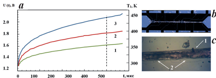
Рис. 5. а – Осциллограммы системы Si-диэлектрик-Al при пропускании одиночного импульса тока амплитудой j=3 \cdot 10^{10} А/м 2 и длительностью 450 мкс, толщина Al-слоя h_1=5 мкм, диэлектрика – h_2=0.1 мкм: 1 – h_2=0 ; 2 – Si 3 N 4 ; 3 – SiO 2 . б – Фрагмент тестовой структуры Al-SiO 2 -Si после прохождения прямоугольного импульса тока j=8 \cdot 10^{10} А/м 2 и длительностью \tau=500 мкс. в – Фотография структуры Al-SiO 2 -Si после прохождения прямоугольного импульса тока j=6 \cdot 10^{10} А/м 2 и длительностью \tau=400 мкс: 1 – дорожка металлизации; 2 – микротрещины пленки SiO 2 .
