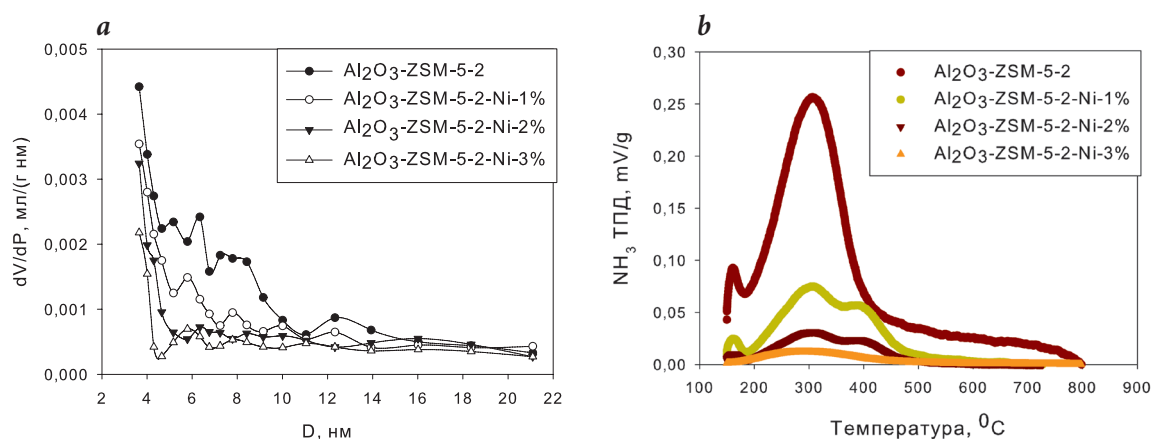
Рис. 5. а – Распределение пор по размерам и б – кривые температурнопрограммируемой десорбции аммиака для Ni-модифицированных мембран.
