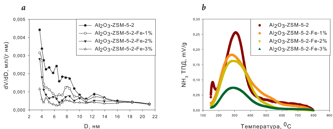
Рис. 4. а – Распределение пор по размерам и б – кривые температурнопрограммируемой десорбции аммиака для Fe-модифицированных мембран.
