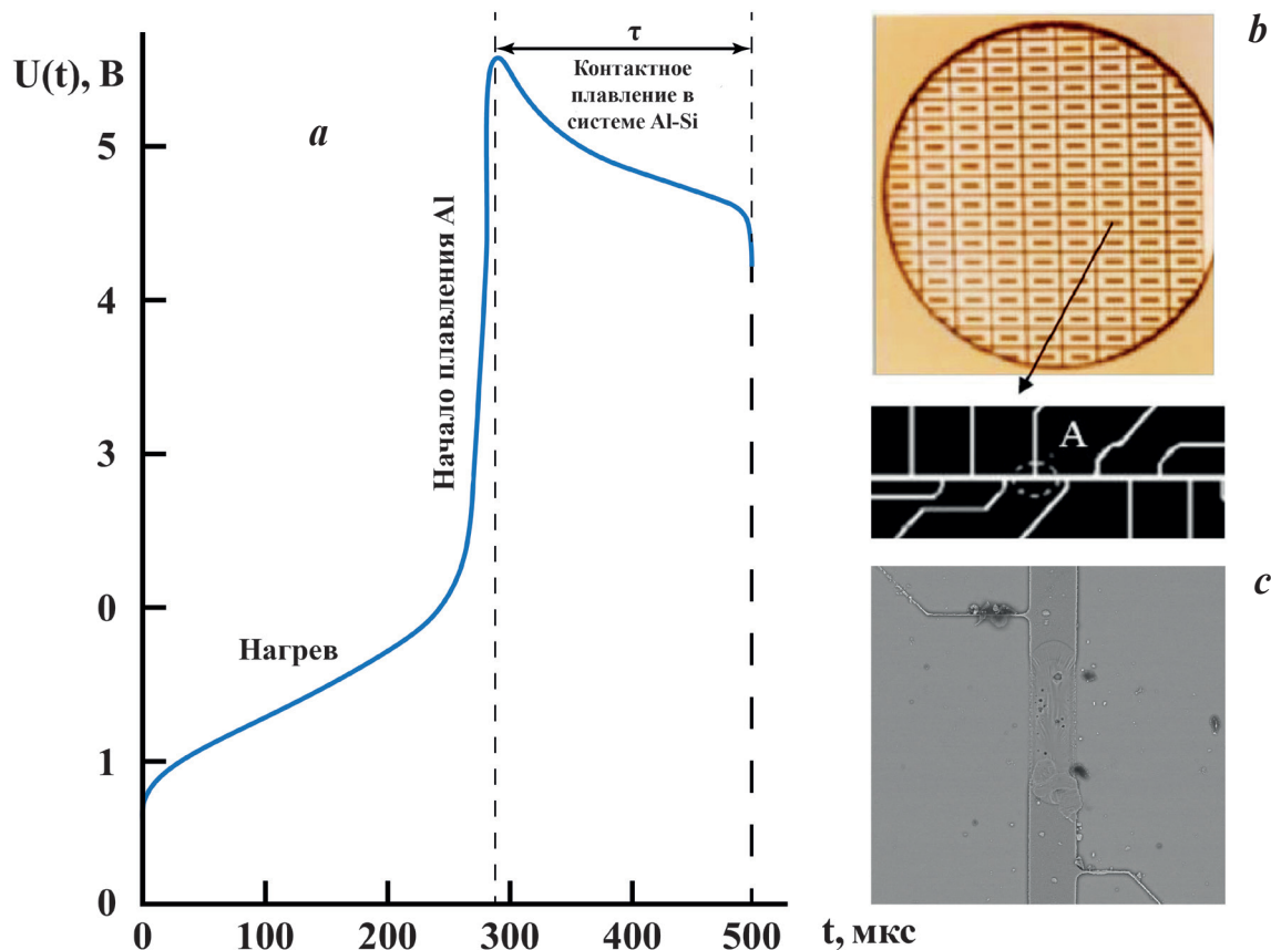
Рис. 1. а – Осциллограмма U(t) при прохождении одиночного импульса тока амплитудой j = 5.8 \cdot 10^{10} А/м 2 , длительность импульса \tau = 500 мкс, через алюминиевую дорожку металлизации, лежащую на Si. Толщина алюминиевой пленки – 3 мкм, длина и ширина – 5 мм и 50 мкм соответственно, толщина кремниевой подложки – 1 мм. Зона \tau – время контактного плавления. б – Вид тестовых структур; в – РЭМ-структуры Al-Si после прохождения прямоугольного импульса тока.
