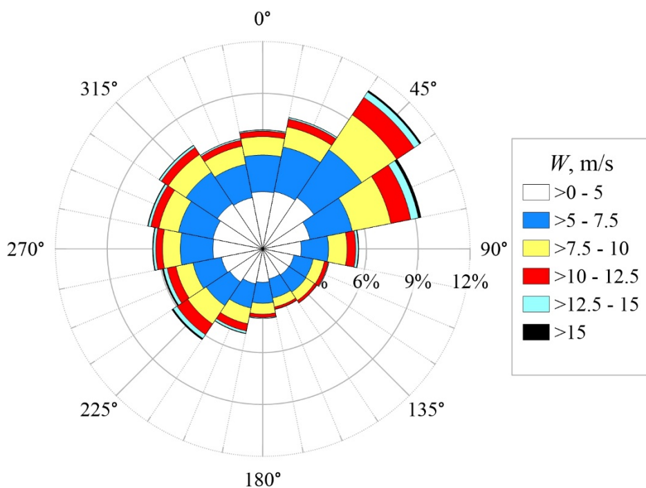
Fig. 8. Wind rose
