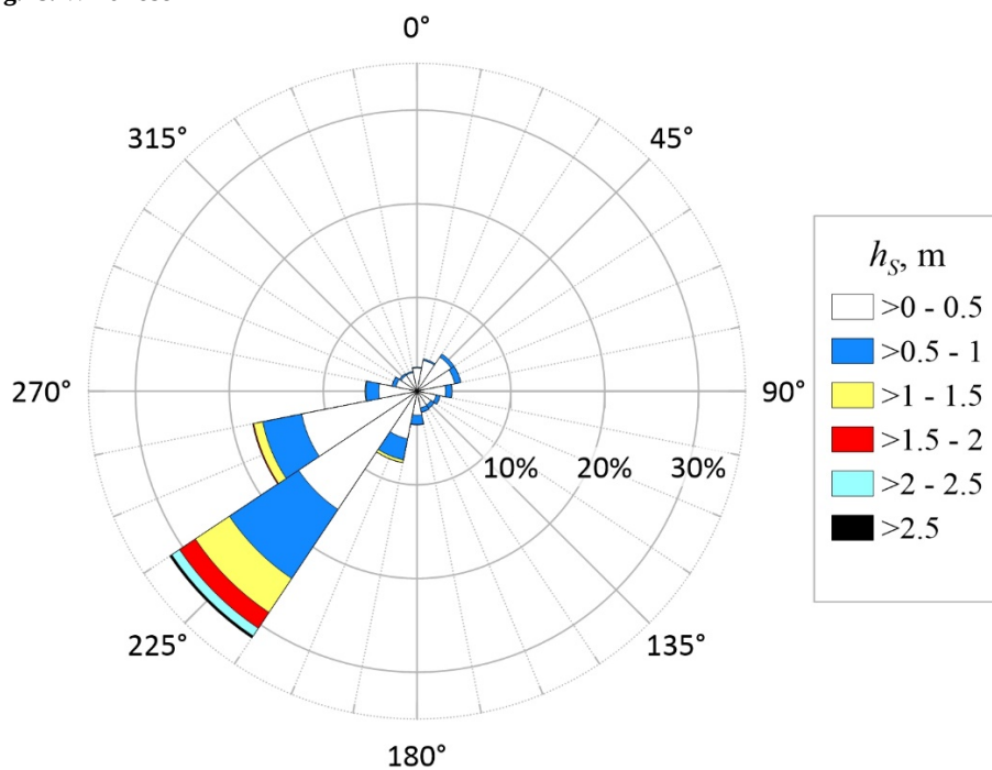
Fig. 9. Wave rose
