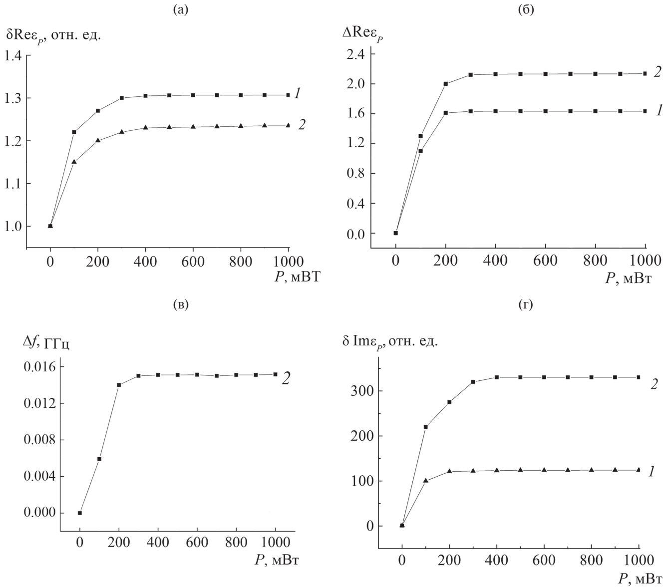
Рис. 1. Измеренная в волноводном резонаторе (4.7 ГГц) динамика диэлектрической проницаемости Si (1) и GaAs (2) в зависимости от мощности оптического облучения P (на длине волны \lambda = 0.97 мкм) относительно P = 0 : а – \delta \text{Re} \epsilon_p ; б – \Delta \text{Re} \epsilon_p ; в – \Delta f ; г – \delta \text{Im} \epsilon_p .
