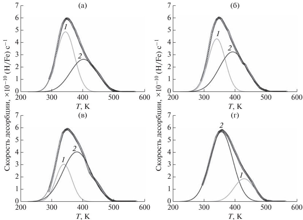
Рис. 4. Аппроксимация гауссианами (сплошные линии, 1–2) спектра термодесорбции водорода [44] (точки), полученного при скорости нагрева \beta = 6.66 К/мин для образцов железа, подвергнутых электрохимическому наводороживанию после холодной пластической деформации растяжением, степень деформации \varepsilon = 0 (а); 5 (б); 10 (в); 15% (г).
