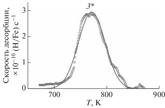
Рис. 5. Аппроксимация гауссианом (сплошная линия, 1) спектра термодесорбции водорода [44] (точки), полученного при скорости нагрева \beta = 6.66 К/мин для недеформированного образца ПНП-стали, не подвергнутого электрохимическому наводороживанию (в табл. 3 отмечен *).
