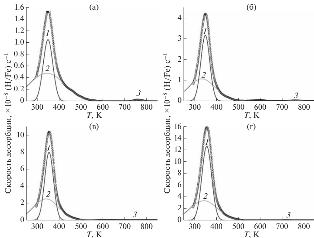
Рис. 3. Аппроксимация гауссианами (сплошные линии, 1–3) спектра термодесорбции водорода [44] (точки), полученного при скорости нагрева \beta = 6.66 К/мин для образцов ПНП-стали, подвергнутых электрохимическому наводороживанию после холодной пластической деформации растяжением, степень деформации \varepsilon = 0 (а); 5 (б); 10 (в); 15% (г).
