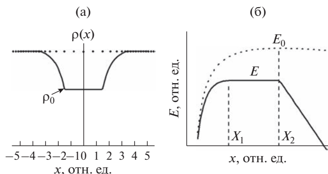
Рис. 1. Иллюстрация флуктуационного разрежения (а) в распределении атомов раствора r(x) = \rho(x)/\rho , приводящего к понижению потенциального барьера для образования пары кинков (б). Пунктирной линией показан потенциал пары кинков при однородном распределении атомов раствора в ядре дислокации.
