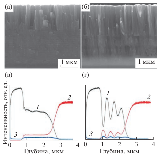
Рис. 1. РЭМ-изображения поперечного сечения покрытий на подложках из Si(110) и профили распределения Cr (1), Zr (2) и O (3) по глубине распыления покрытий ZrO_2/Cr-50 (а, в) и ZrO_2/Cr-250 (б, г) на подложке из сплава Э110.
