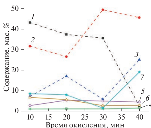
Рис. 3. Фазовый состав образца с покрытием ZrO_2/Cr-250 в зависимости от времени окисления: 1 — Cr; 2 — Cr_2O_3 ; 3 — моноклинная фаза ZrO_2 ; 4 — тетрагональная фаза ZrO_2 ; 5 — ZrN; 6 — Zr; 7 — Cr_2N .
