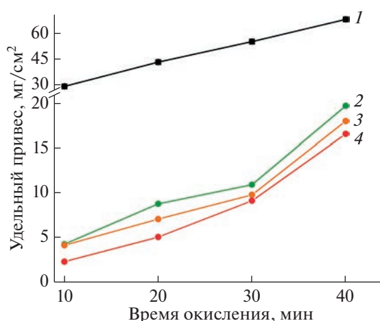
Рис. 2. Привес образцов из сплава Э110 без покрытия (1) [18], с однослойным Cr (2) [18] и многослойными покрытиями ZrO_2/Cr-50 (3) и ZrO_2/Cr-250 (4) после окисления на воздухе.
