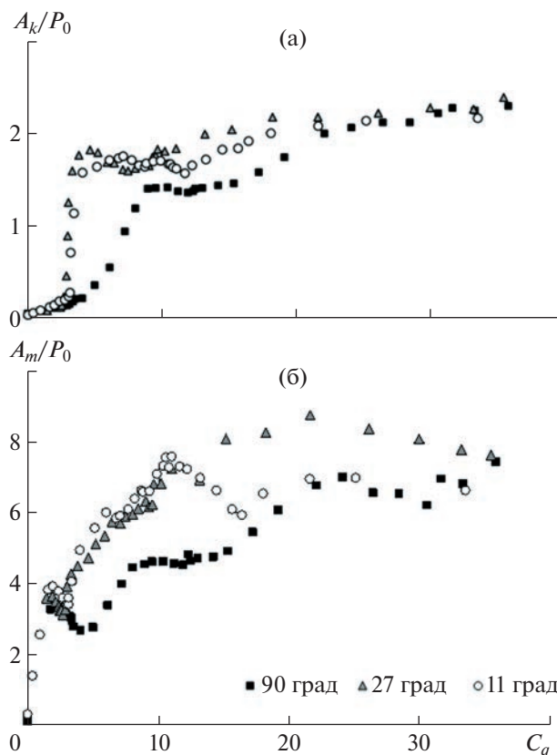
Рис. 10. Зависимость относительной интенсивности пульсаций давления в каверне (а) и ударных импульсов давления на экране (б) от коэффициента поддува для тех же условий, что и на рис. 9.
