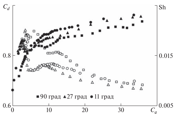
Рис. 9. Зависимость C_d от C_q (левая шкала, залитые знаки) и Sh от C_q (правая шкала, прозрачные знаки) для сопла длиной 55 мм (кривая 1 на рис. 6) при наличии перед кавитатором линейного конфузора с углами сужения 90°, 27°, 11°.
