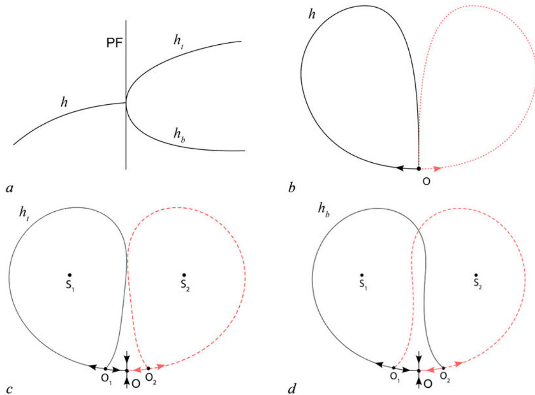
Рис. 8. Бифуркация седлового состояния равновесия с парой гомоклинических траекторий [25, 26]. a — Бифуркационная диаграмма: h , h_t — гомоклинические бифуркации, PF — бифуркации «вилка», h_b — гетероклиническая бифуркация. b — Гомоклиническая «восьмерка-бабочка» на кривой h , c — петля сепаратрисы для O_1 ( O_2 , по симметрии) на кривой h_t , d — гетероклинический контур между O_1 и O_2 на кривой h_b (цвет онлайн)
