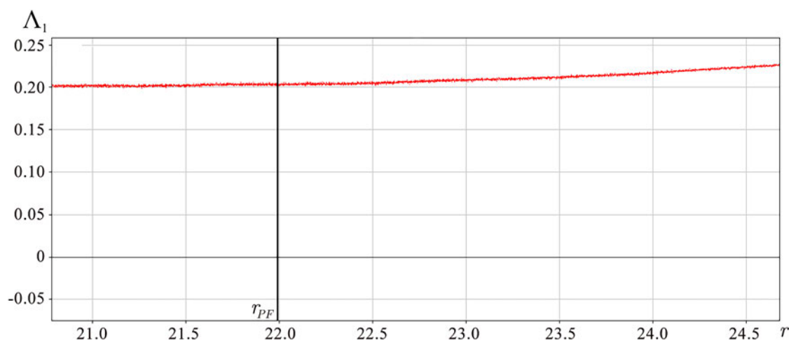
Рис. 5. График зависимости максимального показателя Ляпунова в системе (2), построенный по 10^4 точкам вдоль маршрута p_1p_2 : \sigma = 3, r \in [20.65, 24.7] . В точке r = r_{PF} \approx 22 седловое состояние равновесия O , входящее в аттрактор Лоренца, претерпевает бифуркацию «вилка», что, однако, не сказывается на монотонной зависимости показателя Ляпунова от параметра. Этот эксперимент свидетельствует о возможной псевдогиперболичности исследуемых хаотических аттракторов (цвет онлайн)
