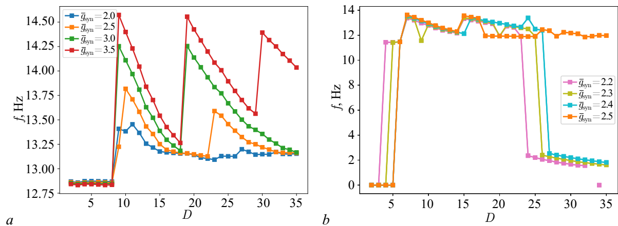
Рис. 7. Зависимость частоты колебаний в кольце f от количества нейронов в сети D при разных значениях синаптической проводимости g_{syn} для нейронов, расстроенных по параметрам. w = 100 мс. Проводимость утечки: g_L = 0.043 мкСм. Фрагмент (а) построен для нейронов, находившихся в бистабильном режиме, фрагмент (б) построен для нейронов, находившихся в чисто возбудимом режиме с единственным аттрактором в виде устойчивого фокуса (цвет онлайн)
