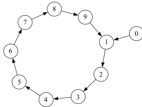
Рис. 1. Структура рассматриваемой сети из нейронов гиппокампа. Нейрон №0 используется только для запуска колебательной активности и в генерации ритма непосредственно не участвует
