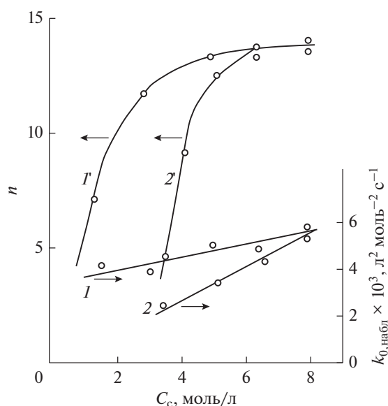
Рис. 3. Зависимости k_{0, \text{набл}} и параметра n от средней концентрации пентанола-1 в пара-ксилоле (1,1') и 1,4-диоксана (2,2') при 100°C.
