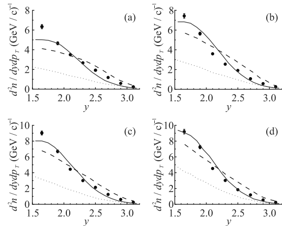
Рис. 2. (Цветной онлайн) Распределения \pi^+ мезонов по быстротам с 0.1 \leq p_T \leq 0.2 ГэВ/с в соударениях ^{40}\text{Ar} + \text{Al} (a), Cu (b), Sn (c), Pb (d) при E_{\text{lab}} = 3.2 А · ГэВ. Точки – экспериментальные данные BM@N коллаборации [14] без учета систематических ошибок. Сплошные кривые – расчеты по новой модели Geant4 FTF. Штриховые линии – расчеты по модели DCM [15], выполненные коллаборацией. Пунктирные кривые – расчеты по старой модели Geant4 FTF
