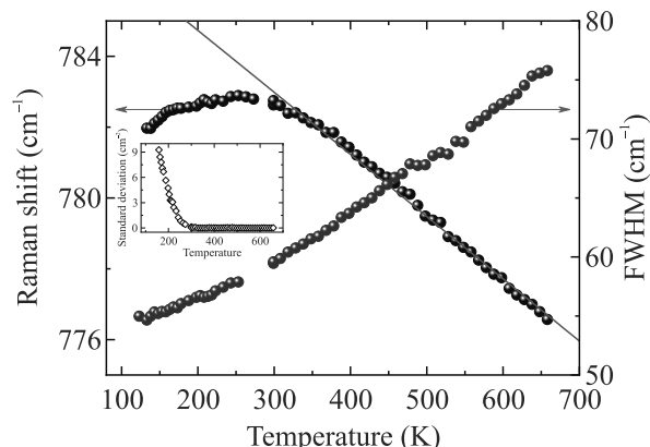
Рис. 3. (Цветной онлайн) Температурная зависимость частоты и ширины на полувысоте (FWHM) моды D ( \nu_2 = 781 \text{ см}^{-1} ) в рамановских спектрах PNN с VV поляризацией. Сплошная линия – результат аппроксимации экспериментальных данных выражением (3) (см. текст). На вставке показана температурная зависимость отклонения экспериментальных данных от расчетной зависимости частоты согласно выражению (3)
