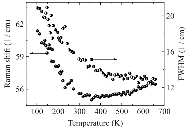
Рис. 5. Температурные зависимости частоты (а) и ширины на полувысоте (FWHM) (b) моды A ( \nu_4 = 55 \text{ см}^{-1} ) в рамановских спектрах PNN с VH поляризацией
