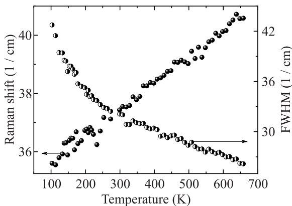
Рис. 4. Температурные зависимости частоты и ширины на полувысоте (FWHM) моды B ( \nu_3 = 37 \text{ см}^{-1} ) в рамановских спектрах PNN с VH поляризацией
