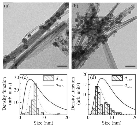
Рис. 2. (Цветной онлайн) ПЭМ-микрофотографии образцов (\text{Mg}_{1-x}\text{Co}_x)_3\text{Si}_2\text{O}_5(\text{OH})_4 (а) x = 0.6 и (b) x = 1 после частичного восстановления в атмосфере аргон-водорода при 550^\circ\text{C} , микронмаркер равен 50 нм; распределения частиц по размерам по данным ПЭМ ( d_{\text{TEM}} , столбцы и пунктирная линия) и распределение кристаллитов по размерам по данным порошковой рентгеновской дифрактометрии ( d_{\text{XRD}} , сплошная линия) по пику (111) для образцов (c) x = 0.6 и (d) x = 1
