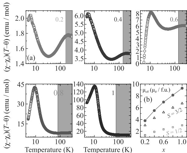
Рис. 4. (Цветной онлайн) (a) – Температурные зависимости (\chi - \chi_0)(T - \theta) ( T \in [4; 300] К) для каждого состава (\text{Mg}_{1-x}\text{Co}_x)_3\text{Si}_2\text{O}_5(\text{OH})_4 ( x = 0.2, 0.4, 0.6, 0.8, 1 ) в логарифмическом масштабе, серым цветом обозначен диапазон обработки данных по модифицированному закону Кюри-Вейсса и (b) концентрационная зависимость экспериментальной (закрашенные круглые символы, соединенные линией) и теоретического (полые треугольные символы для S = 3/2 и полые квадратные символы для S = 1/2 ) эффективного магнитного момента
