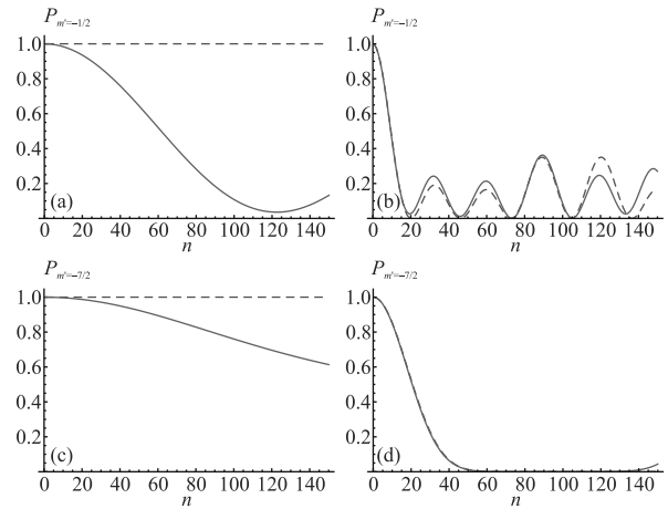
Рис. 2. (Цветной онлайн) Расчеты величины P_{m'} после действия композитной рамсеевской последовательности \{(\pi/2, -\pi/2)^n, \pi\} для \kappa = 0 (красная штриховая линия) и \hbar\kappa/\Omega_{\text{rf}} = 0.00004 (зеленая сплошная линия): (a) — P_{m'=-\frac{1}{2}} на основе резонансного гамильтониана (9); (b) — P_{m'=-\frac{1}{2}} на основе полного гамильтониана (3) [или (7)] с использованием Фурье-анализа; (c) — P_{m'=-\frac{7}{2}} на основе резонансного гамильтониана (9); (d) — P_{m'=-\frac{7}{2}} на основе полного гамильтониана (3) [или (7)] с использованием Фурье-анализа. Параметры расчетов: \Omega_{\text{rf}}\tau = \pi , \Omega_L/\Omega_{\text{rf}} = 100 , \delta = 0 , \tau_R = 10\tau
