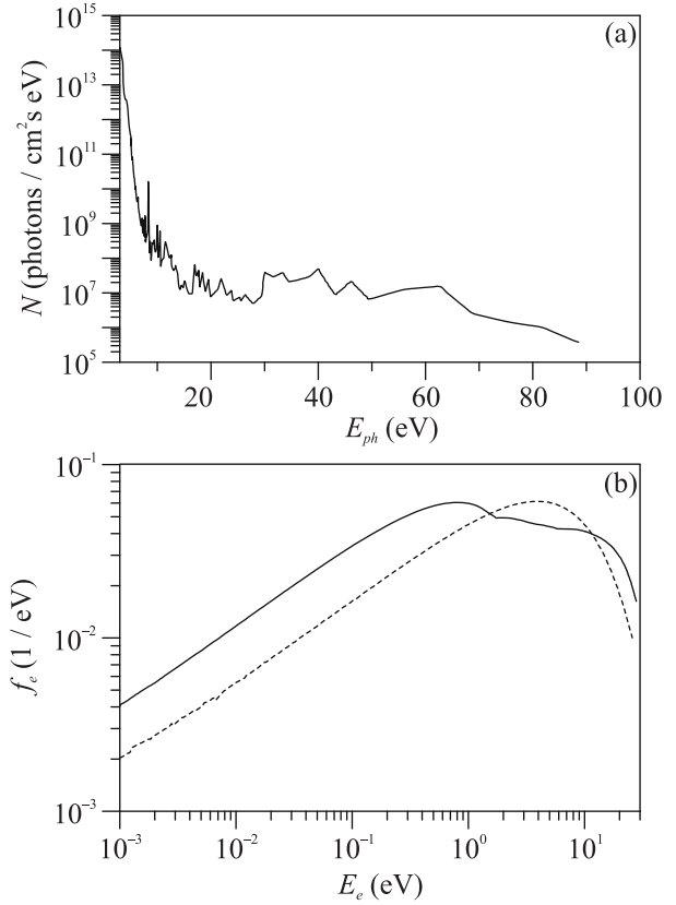
Рис. 1. Потоки солнечного излучения на орбите Сатурна в зависимости от энергии фотонов (в логарифмическом масштабе), соответствующие солнечному максимуму (а). Функция распределения фотоэлектронов f_e по энергиям (сплошная кривая) у освещенной части поверхности Энцелада, соответствующая солнечному максимуму, и максвелловское распределение (пунктирная кривая), вычисленное для значений средней энергии фотоэлектронов, характеризующих распределение, изображенное сплошной кривой (б)
