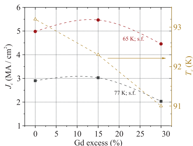
Рис. 3. (Цветной онлайн) Зависимость критического тока и температуры сверхпроводящего перехода в ВТСП – 2 ленты с разным содержанием Gd
