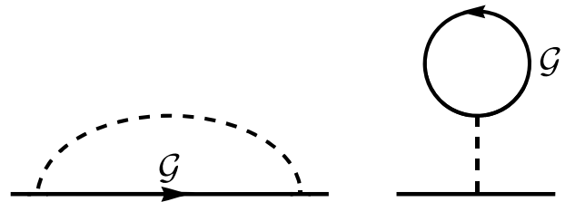
Рис. 1. Диаграммы типа Фока и Хартри для собственной энергии в самосогласованном борновском приближении. Сплошные линии обозначают самосогласованные функции Грина, а штрихованные показывают взаимодействие, индуцированное диссипацией (функции Грина бозона \mathcal{D}_{\mathbf{p},\mathbf{a},\alpha}(\omega) )
