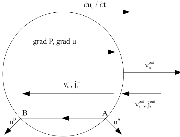
Рис. 1. При движении шарика аэрогеля со скоростью \frac{\partial u_0}{\partial t} в сверхтекучем ^3\text{He} внутри объема, занимаемого аэрогелем, создается градиент давления и химического потенциала жидкости в направлении движения. Согласно уравнению сохранения сверхтекучей скорости это приводит к возникновению сверхтекучего потока в противоположном направлении. Из закона сохранения суммарного импульса системы при появлении данного движения на аэрогель начинает действовать дополнительная сила вдоль направления движения, увеличивающая итоговую частоту колебаний
