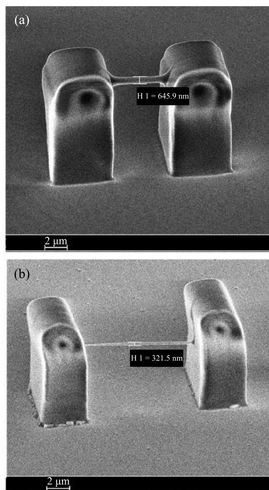
Рис. 2. СЭМ изображение калибровочной структуры, состоящей из двух пьедесталов и перемычки (нити) между ними длиной 10 мкм, напечатанной в один проход движения перетяжки лазерного излучения: (а) – в отсутствие пространственного фильтра в пучке накачки, поперечные размеры нити (ширина и высота) составили 660 \times 690 \text{ нм} ; (б) – в присутствии пространственного фильтра, поперечные размеры нити 250 \times 325 \text{ нм}
