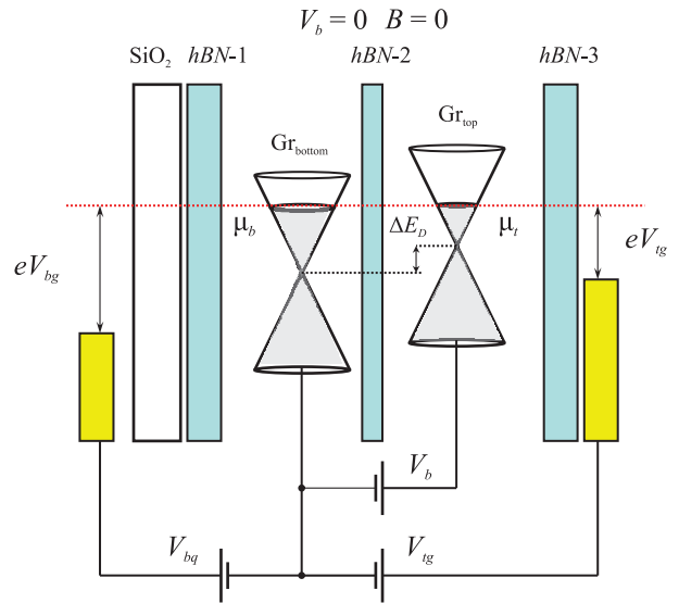
Рис. 1. (Цветной онлайн) Схема равновесного туннелирования между монослоями графена, где конусами Gr top и Gr bottom обозначены верхний и нижний монослои графена, hBN-1, hBN-2 и hBN-3 – нижний подзатворный, туннельный и верхний слой нитрида бора соответственно, SiO 2 – основной диэлектрический слой нижнего затвора, μ t и μ b – химические потенциалы в верхнем и нижнем слоях. Энергетический сдвиг дираковских точек, зависящий от V tg , V bq и V b , обозначен как ΔE D
