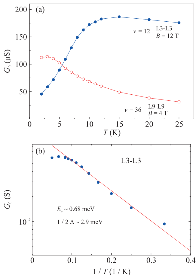
Рис. 5. (Цветной онлайн) (а) – Зависимости G_0 = dI/dV_b при V_b = 0 от температуры для переходов L9-L9 при B = 4 Тл (красная) и L3-L3 при B = 12 Тл (синяя); (б) – Зависимость G_0 при \nu = 12 , B = 12 Тл для перехода L3-L3 от обратной температуры 1/T
