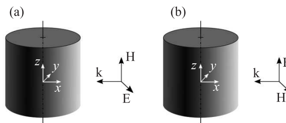
Рис. 2. Взаимная ориентация цилиндра, координатных осей и векторов \mathbf{k} , \mathbf{E} , \mathbf{H} падающей волны. (а) – ТЕ поляризация; (б) – ТМ поляризация [28, 31]
