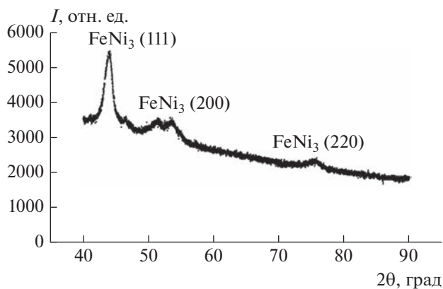
Рис. 2. Рентгенограмма нанопроволок FeNi.
