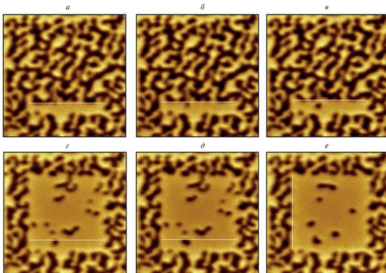
Рис. 1. МСМ изображения доменных структур, снятые после прохода 25-й (а), 27-й (б), 35-й линии (в), 17-й и 18-й линий второй серии (z и д), в конце 9-й серии (е).
