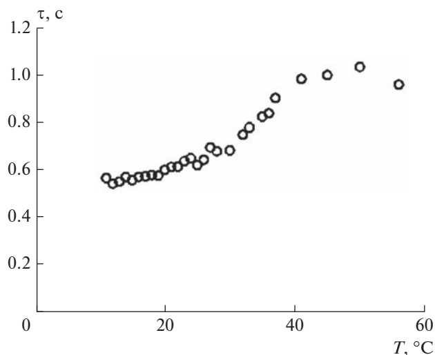
Рис. 4. Температурная зависимость времени релаксации магнитооптического эффекта.
