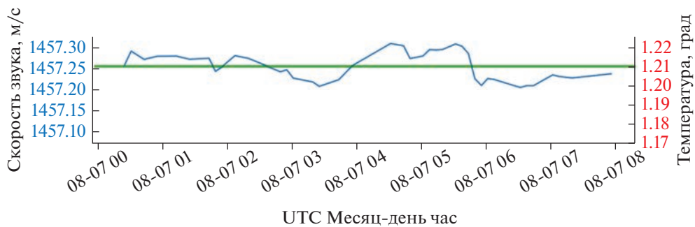
Рис. 6. Скорость звука и температура на оси ПЗК, рассчитанные по последнему приходу акустических сигналов (синий — окно усреднения по часовому интервалу, зеленый — среднее значение по всем измерениям).
