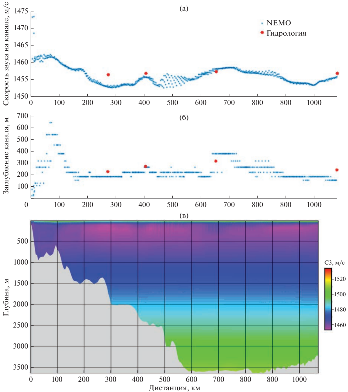
Рис. 3. Данные гибридной гидродинамической модели циркуляции океана NEMO и базы данных земной топографии GEBCO: (а) – изменение скорости звука на оси ПЗК вдоль акустической трассы; (б) – изменение глубины залегания оси ПЗК вдоль акустической трассы; (в) – поле скорости звука и рельеф дна вдоль акустической трассы.
