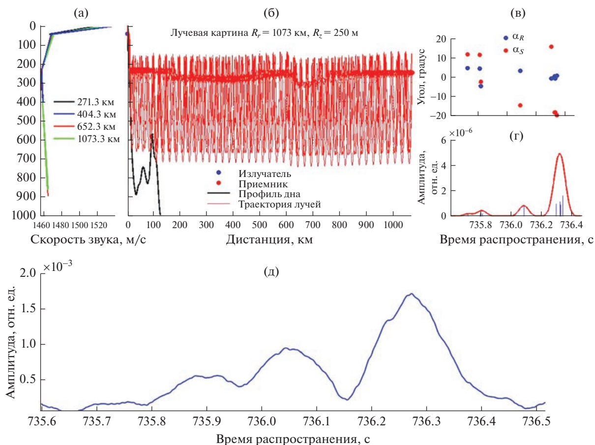
Рис. 7. Результаты моделирования распространения акустических сигналов по трассе длиной 1073 км с использованием программы RAY: (а) – ВРСЗ в точках вдоль трассы; (б) – лучевая картина распространения акустических сигналов для малых углов излучения; (в) – углы выхода и прихода; (г) – модель приходов акустических сигналов и формы импульсных откликов; (д) – экспериментально полученный импульсный отклик для сигнала M127.
