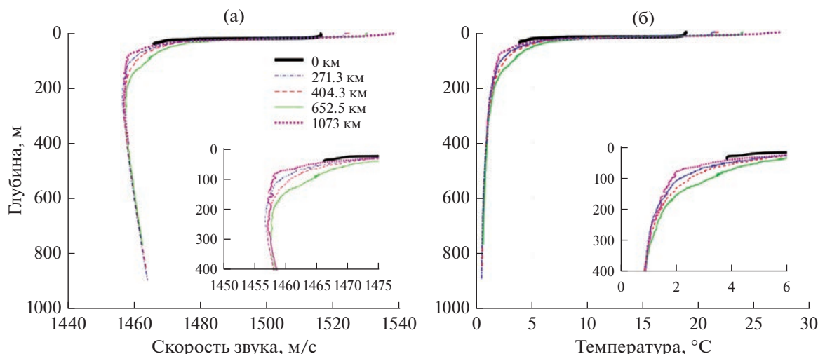
Рис. 2. Измеренные STD-зондом вертикальные распределения (а) — скорости звука и (б) — температуры по глубине в заданных точках. Скорость звука пересчитана косвенно по формуле Чена–Миллера, на основе прямых измерений с датчиков электропроводности, температуры и глубины.
