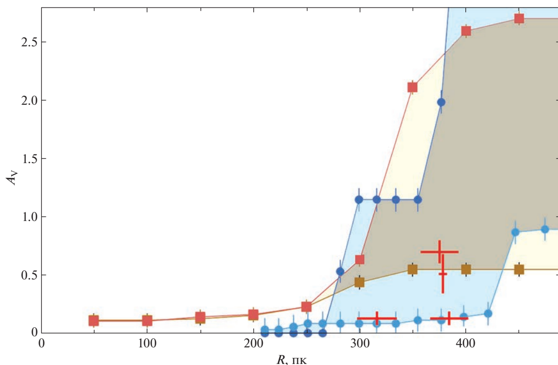
Рис. 14. Зависимость A_V от расстояния в поле зрения скопления NGC 1980, показанная коричневыми квадратами разного оттенка для двух лучей зрения с экстремальными оценками из нашей трехмерной карты, синими кругами разного оттенка для двух лучей зрения с экстремальными оценками из карты GSZ19, красными крестами, размер которых отражает декларируемые авторами неопределенности, для независимых оценок из Кантат-Годэна и др. (2020), Хант, Рефферт (2023) и двух оценок разными методами из Монтейро и др. (2020). Промежуточные оценки из нашей карты и GSZ19 на других лучах зрения в поле NGC 1980 заполняют области, тонированные соответствующим цветом.
