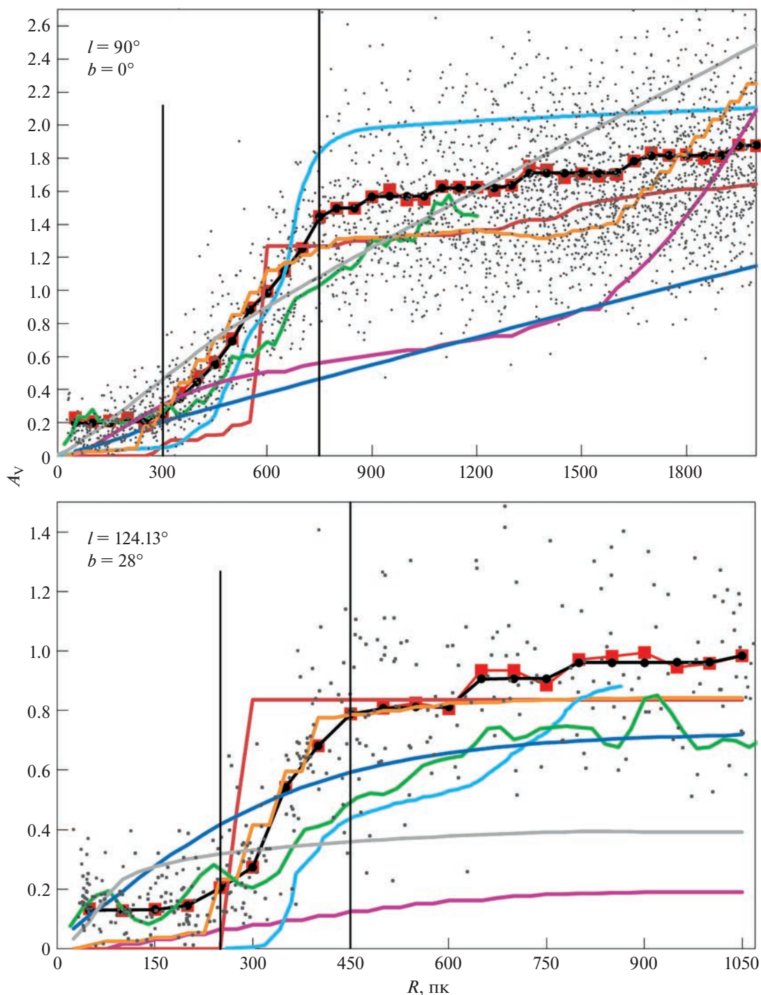
Рис. 7. Поглощение A_V в зависимости от R для двух лучей зрения в направлении облаков Лебедя ( l = 90^\circ , b = 0^\circ ) и Polaris Flare ( l = 124.13^\circ , b = +28^\circ ). Кривыми разного цвета показаны оценки разных карт и моделей: нашей карты до (красный) и после (черный) выравнивания, DCL03 (синий), AL05 (пурпурный), G17 (зеленый), GSZ19 (коричневый), GCU21 (оранжевый), LVB22 (голубой), GMS22 (серый). Отдельными точками показаны использованные нами карлики AKQ22. Вертикальными прямыми показан диапазон расстояний, где происходит существенный рост A_V .
