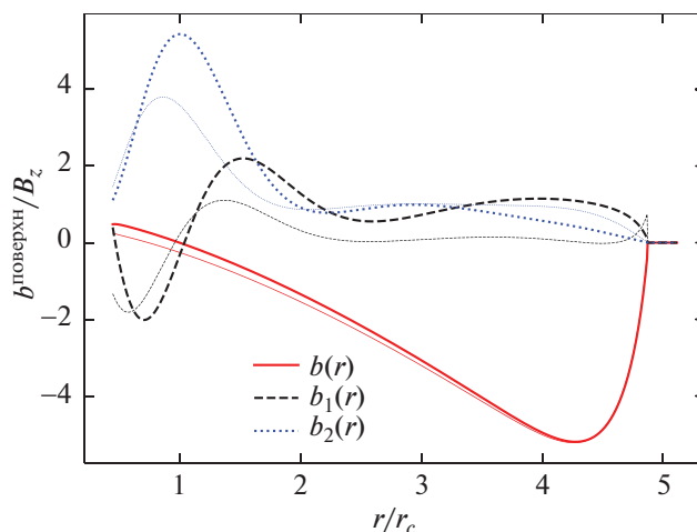
Рис. 3. Сравнение наведенного поля, рассчитанного в цилиндрической системе с использованием алгоритма, описанного в тексте (толстые линии), с полем, рассчитанным в сферической системе численно (тонкие линии того же цвета). Относительная полутолщина диска h_0 = 0.1 , параметр быстроты \omega = 0.3 . Показано поле b и коэффициенты Фурье b_1, b_2 (см. текст) на поверхности диска.
