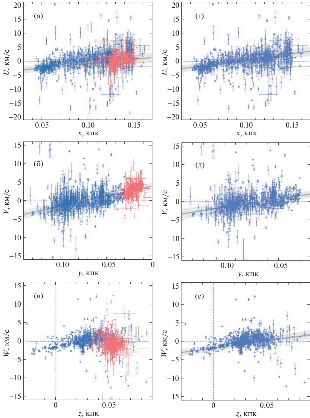
Рис. 8. Скорости U , V , W звезд из ОБ-ассоциации Sco-Cep в зависимости от координат x , y , z .
