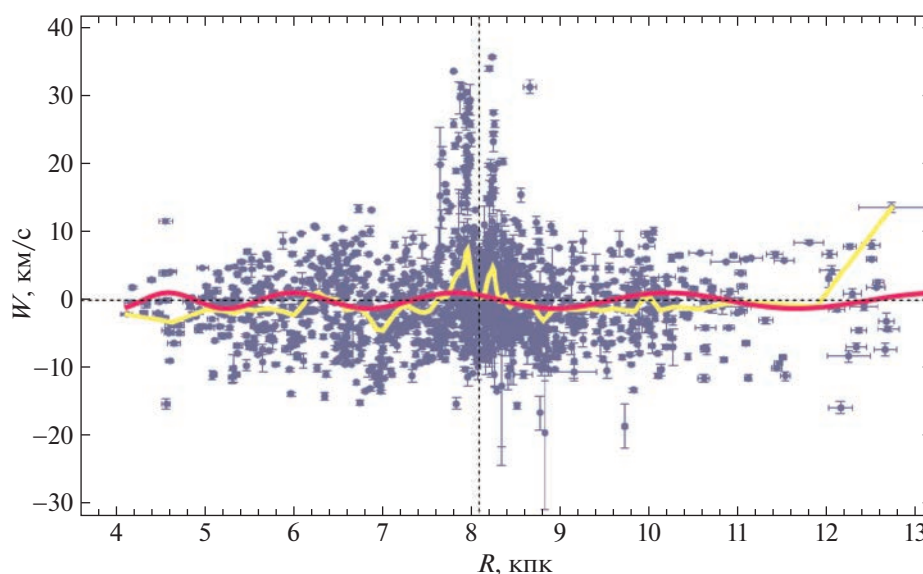
Рис. 1. Вертикальные скорости W в зависимости от галактоцентрического расстояния R выборки РЗС с возрастaми менее 50 млн лет, усредненные данные — желтая линия; периодическая кривая, найденная на основе спектрального анализа — красная линия, рисунок взят из работы Бобылева, Байковой (2023).
